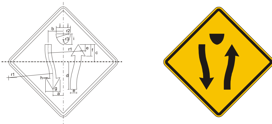
Figura A.114 – Placa A-42a – Início de pista dupla
