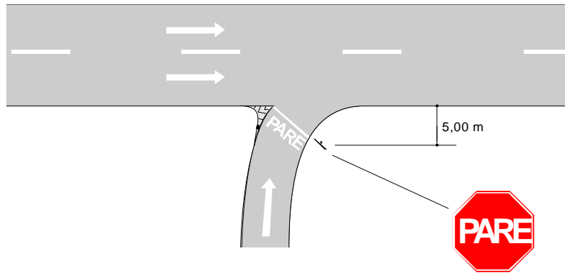
Figura 10 – Aproximação sem ilhas
