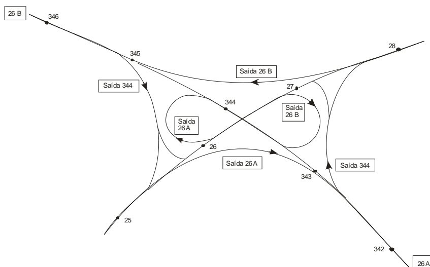
Figura 193 – Acessos múltiplos para uma mesma saída
