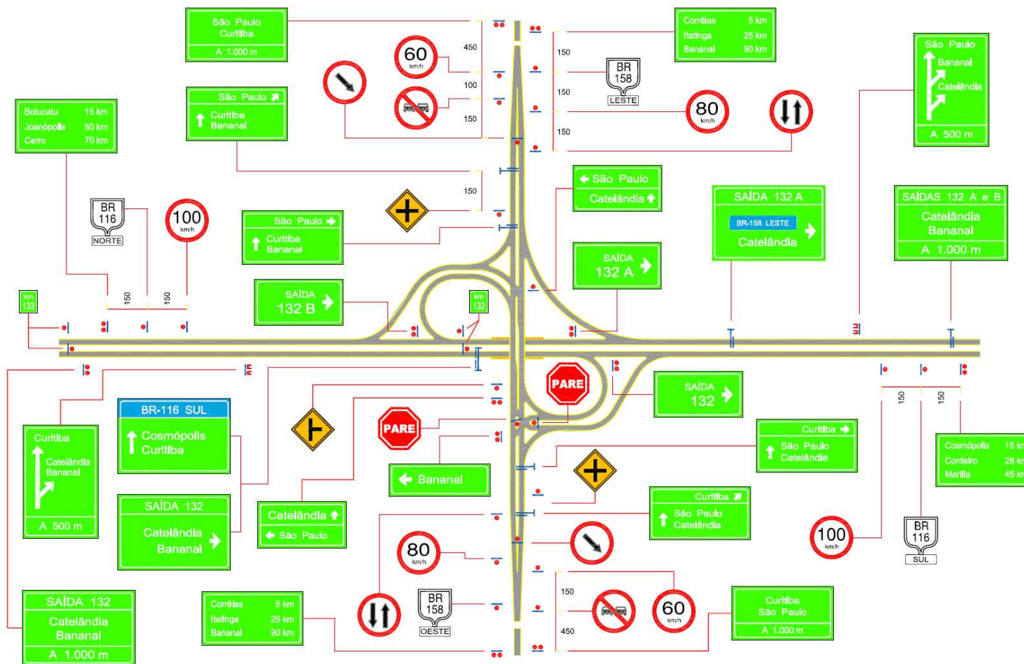
Figura 268 – Interseção em desnível classe I-B com classe I-A
