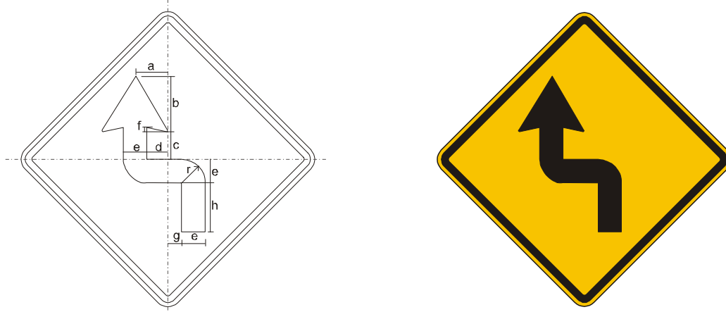
Figura A.61 – Placa A-4a – Curva acentuada em “S” à esquerda
