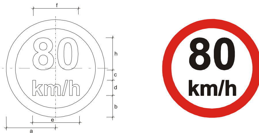
Figura A.26 – Placa R-19 – Velocidade máxima permitida
