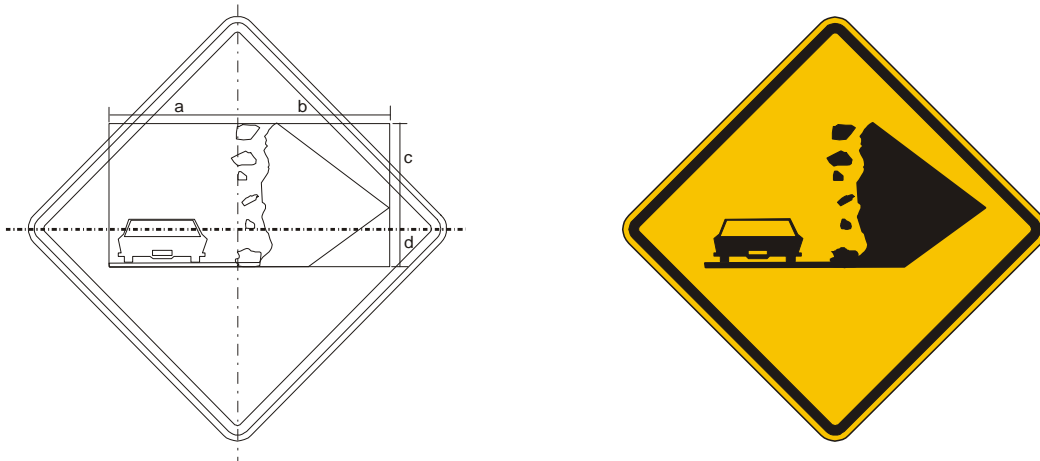
Figura A.95 – Placa A-27 – Área com desmoronamento
