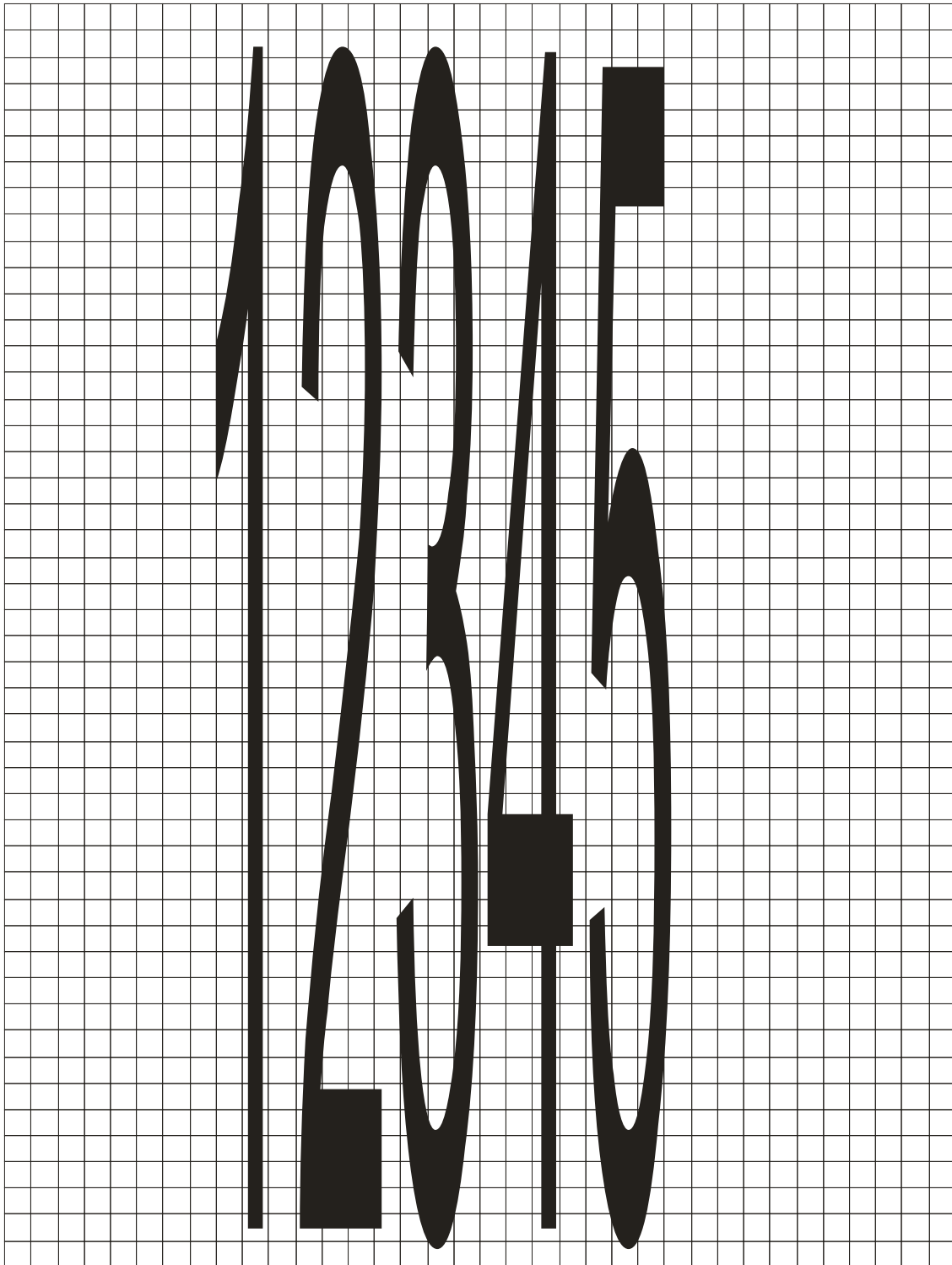
Figura A.159 – Números “1” a “5” – Para V \geq 60 km/h – Vias / trechos rurais
