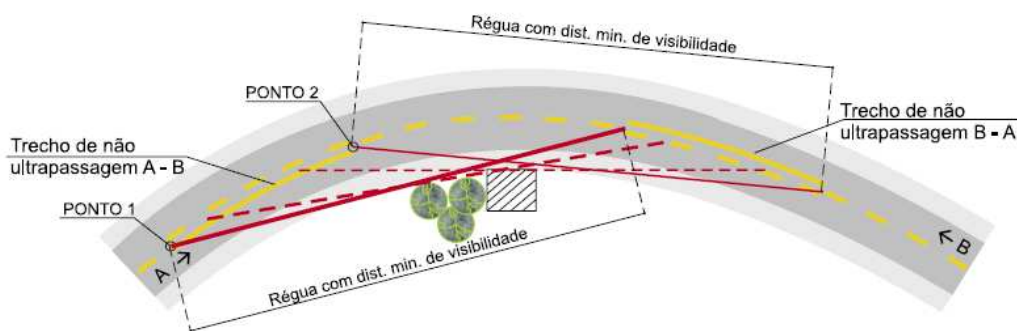
Figura 223 – Distância de visibilidade de ultrapassagem – Horizontal
