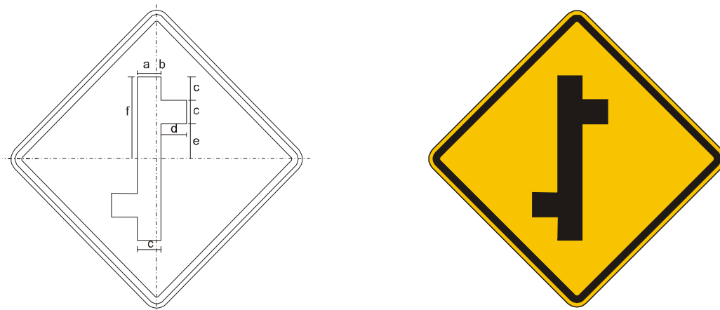
Figura A.72 – Placa A-11a – Junções sucessivas contrárias, primeira à esquerda
