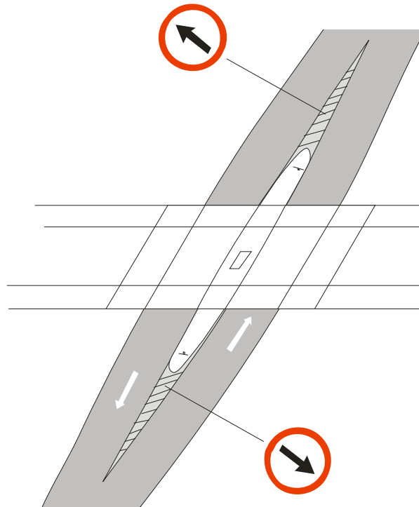
Figura 31 – Ilha de pilar
