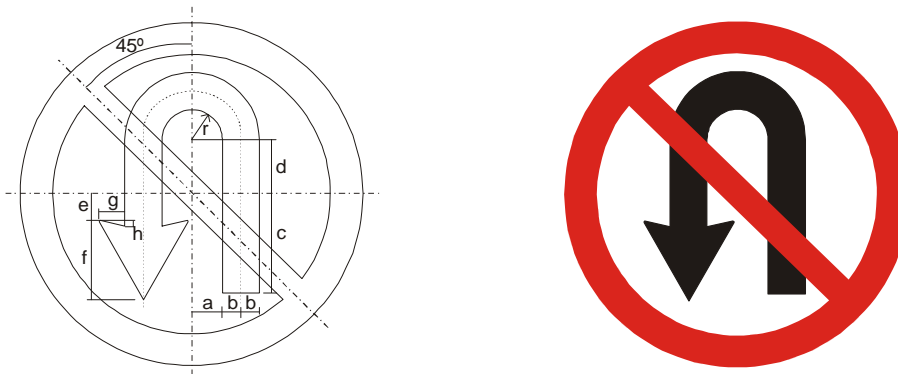
Figura A.8 – Placa R-5a – Proibido retornar à esquerda
