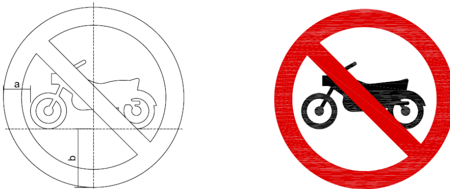
Figura A.50 – Placa R-37 – Proibido trânsito de motocicletas, motonetas e ciclomotores
