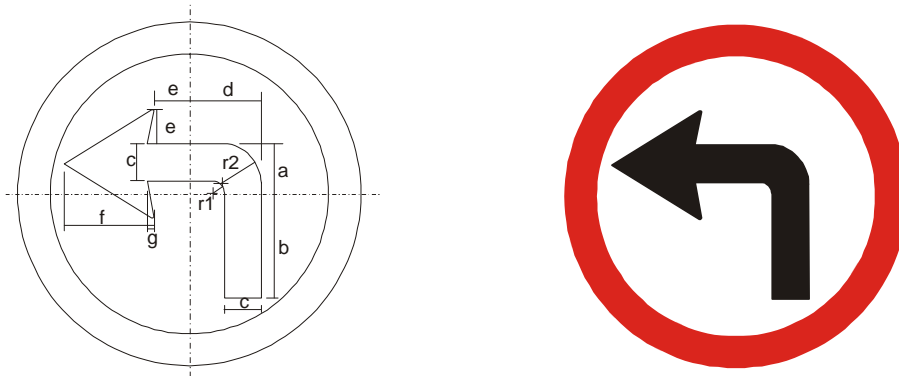
Figura A.33 – Placa R-25a – Vire à esquerda
