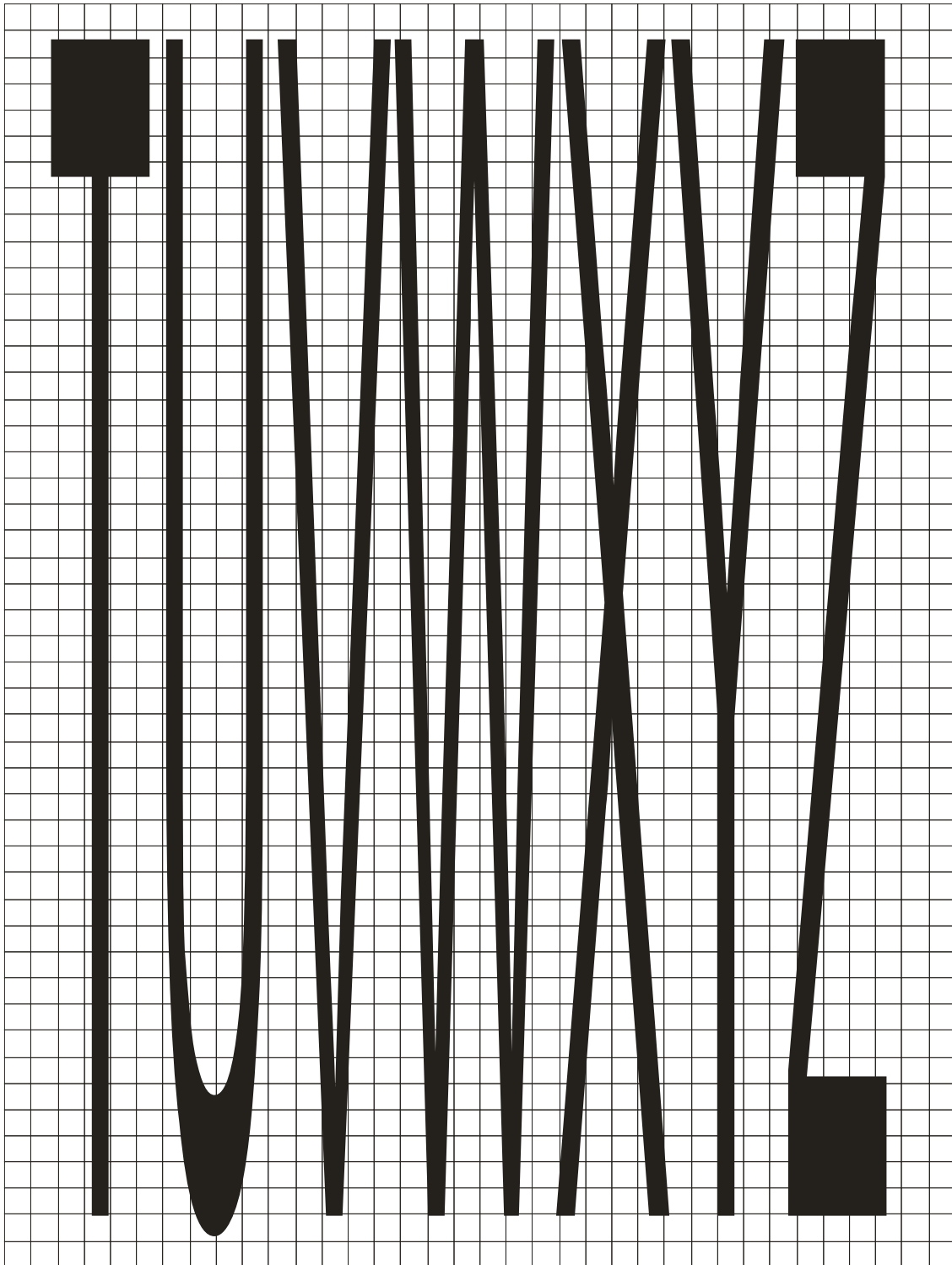
Figura A.158 – Letras T a Z – Para V \geq 60 km/h – Vias rurais
