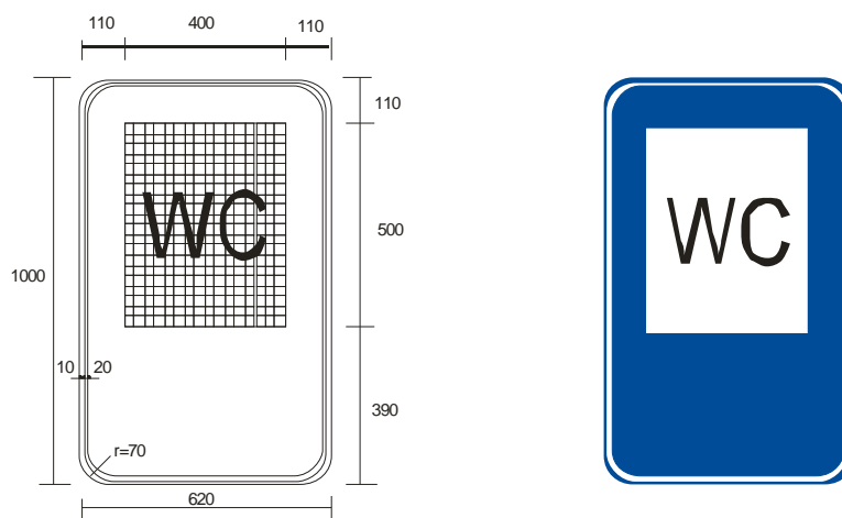
Figura A.125 – Placa I-4 – Serviço sanitário
