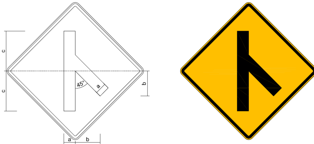
Figura A.76 – Placa A-13b – Confluência à direita
