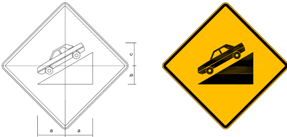
Figura A.83 – Placa A-20a – Declive acentuado
