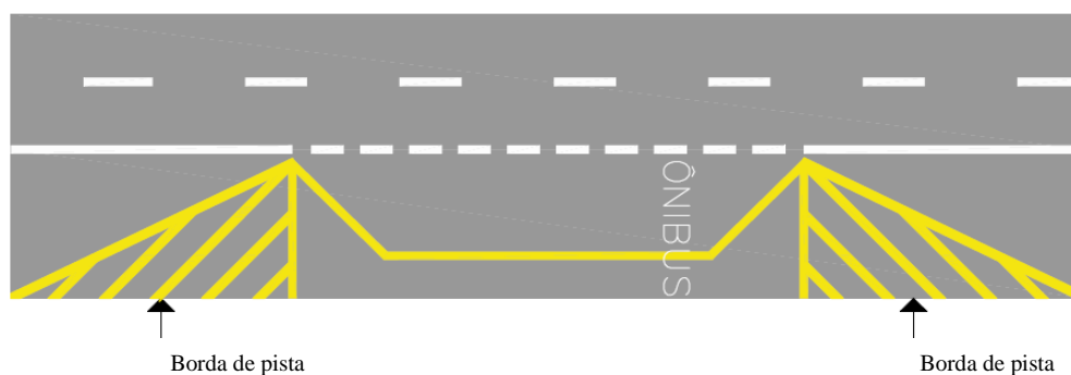
Figura 247 – Modelo de MVE em acostamento de rodovias
