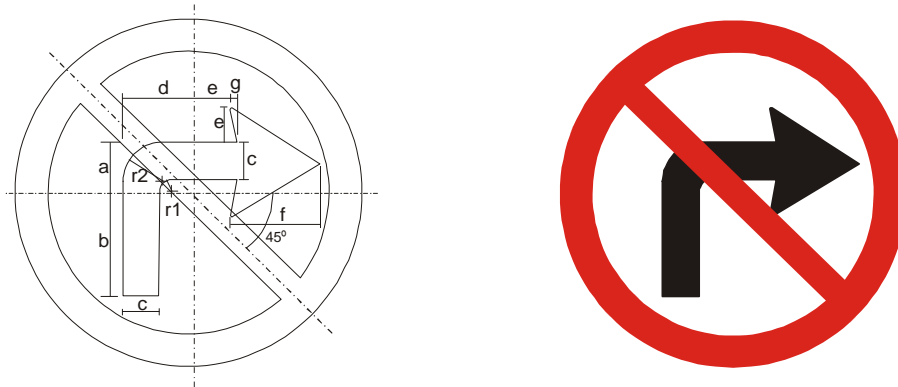
Figura A.7 – Placa R-4b – Proibido virar à direita
