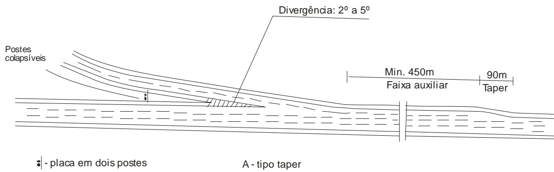
Figura 164 – Pistas divergentes
