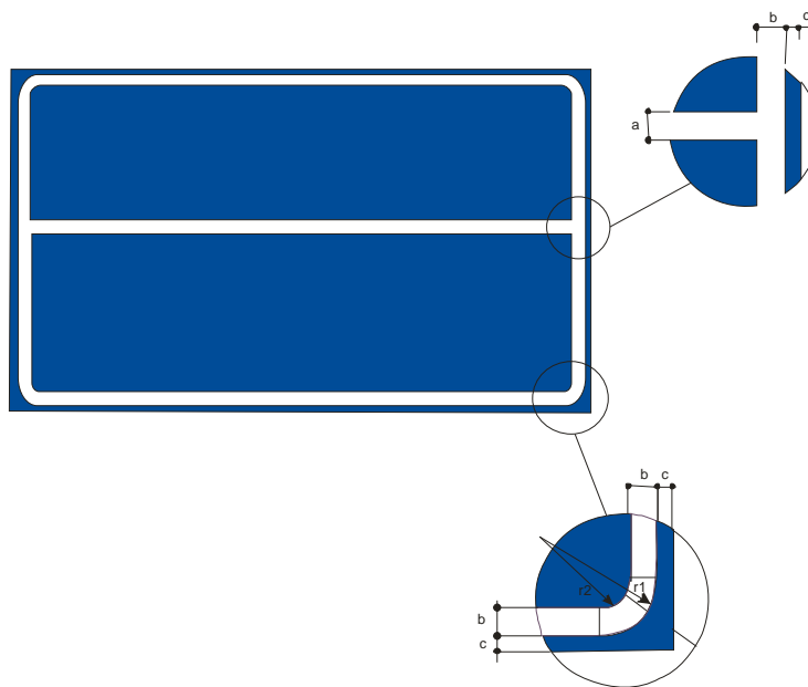
Figura 170 – Desenho da orla e tarja
