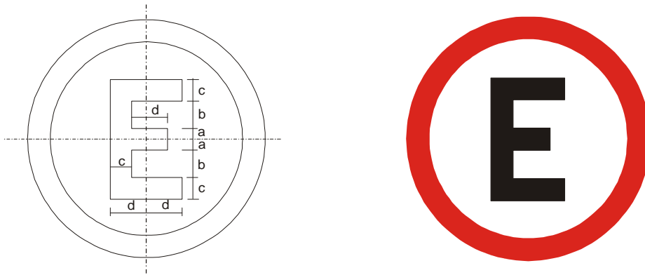
Figura A.11 – Placa R-6b – Estacionamento regulamentado
