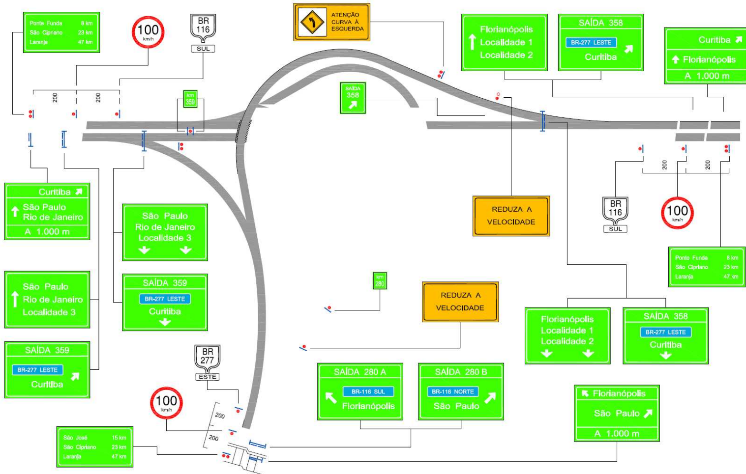
Figura 269 – Interconexão de vias expressas
