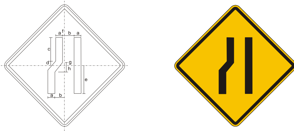
Figura A.86 – Placa A-21b – Estreitamento de pista à esquerda
