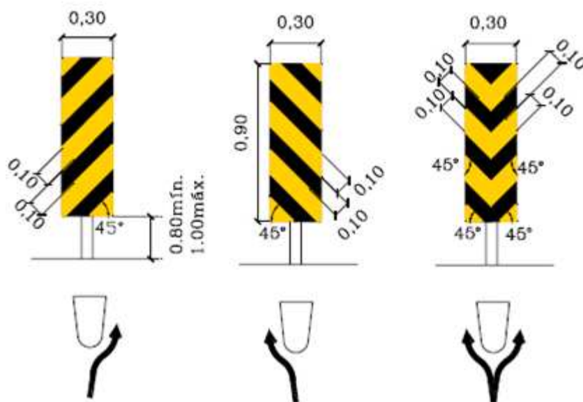
Figura 216 – Marcadores de Perigo
