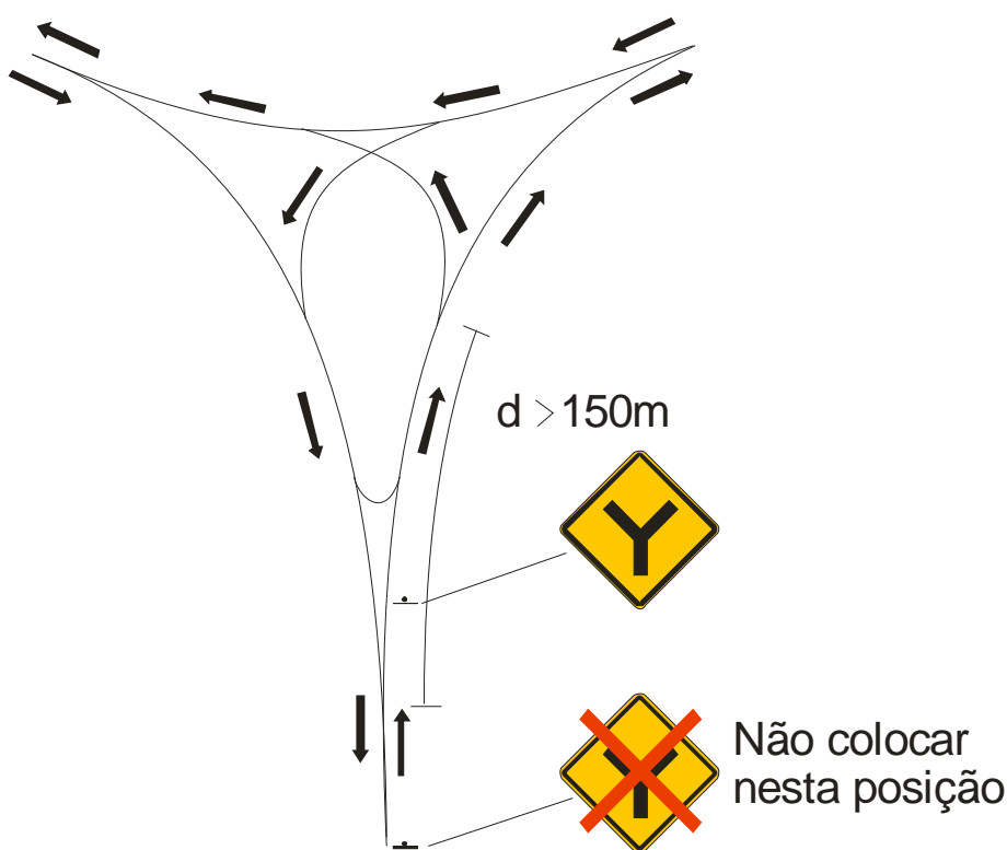
Figura 99 – Interseção em Y
