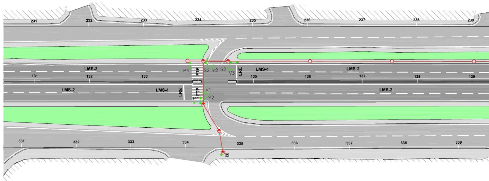
Figura 261 – Projeto de sinalização semafórica
