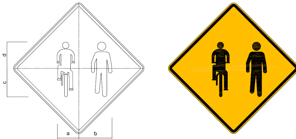
Figura A.100 – Placa A-30c – Trânsito compartilhado por ciclistas e pedestres
