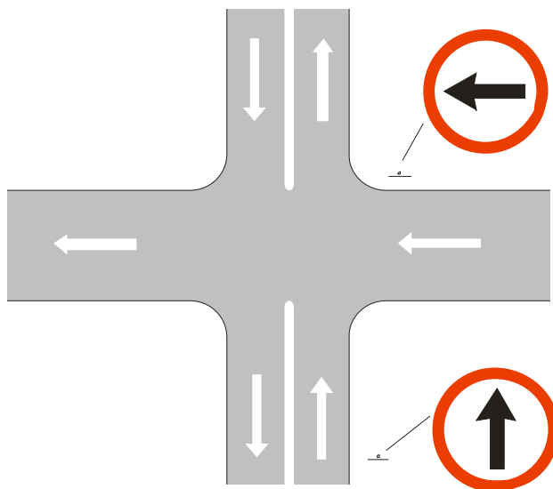
Figura 26 – Cruzamento com pista de mão única correspondente à conversão à esquerda proibida
