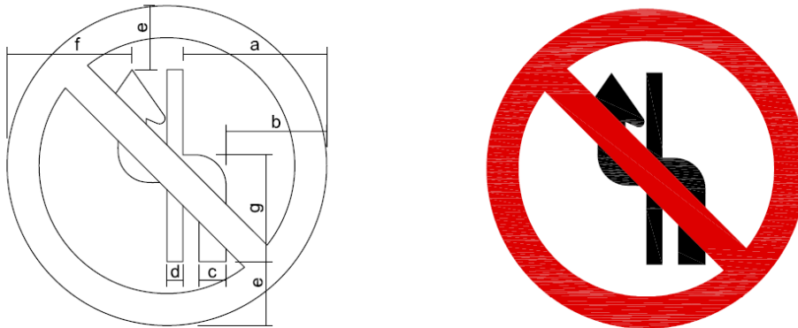
Figura A.15 – Placa R-8b – Proibido mudar de faixa ou pista de trânsito da direita para a esquerda
