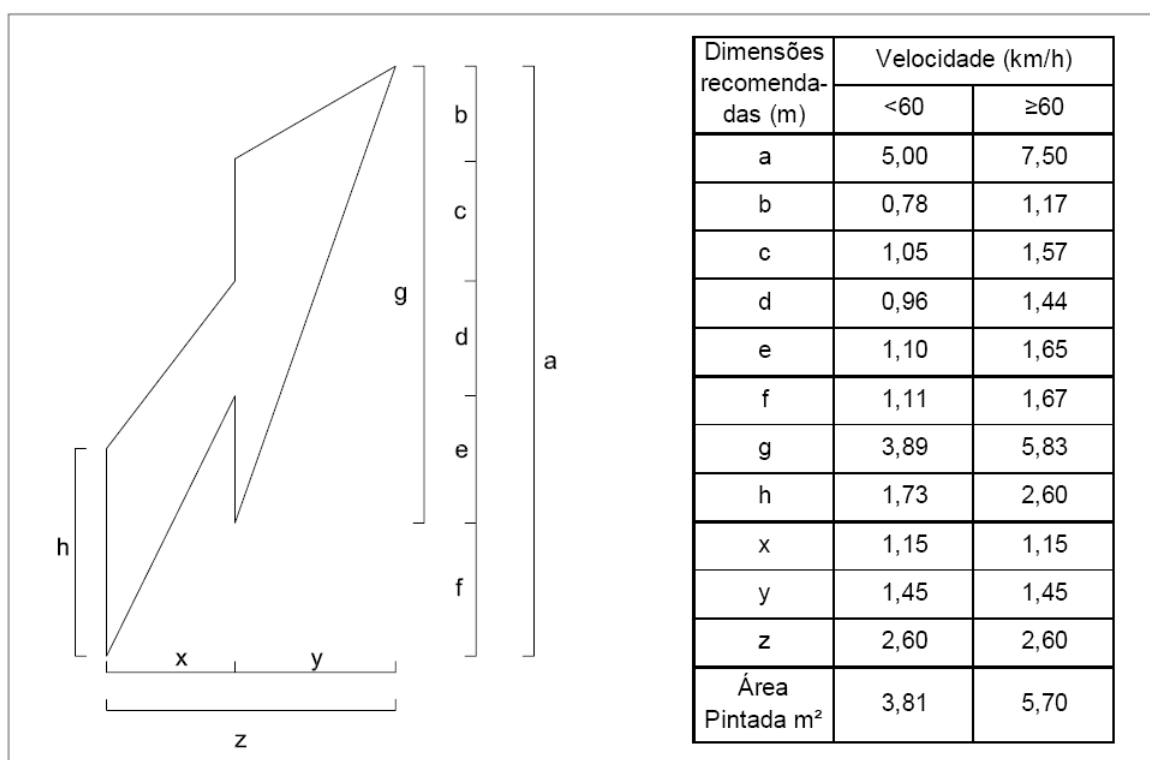
Figura 252 - Seta de mudança obrigatória de faixa (MOF)
