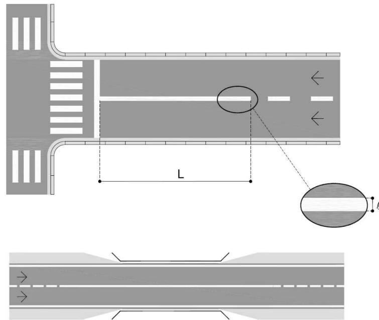
Figura 227 – Linha simples contínua (LMS-1)
