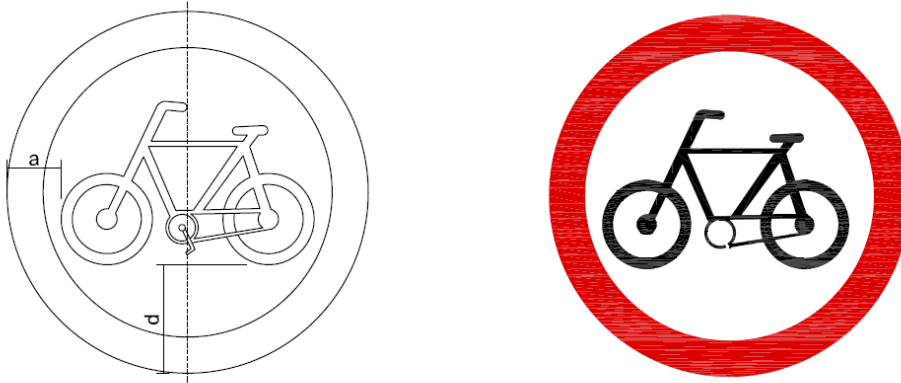
Figura A.45 – Placa R-34 – Circulação exclusiva de bicicletas
