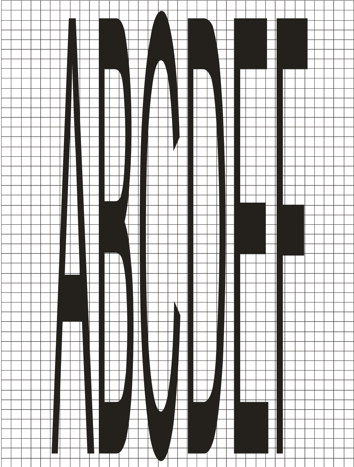
Figura A.155 – Letras A a F – Para V \geq 60 km/h – Vias / trechos rurais
