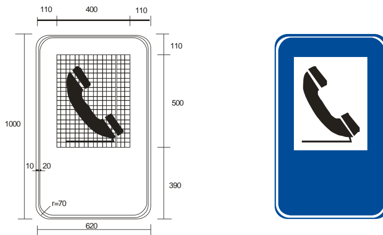
Figura A.124 – Placa I-3 – Serviço telefônico
