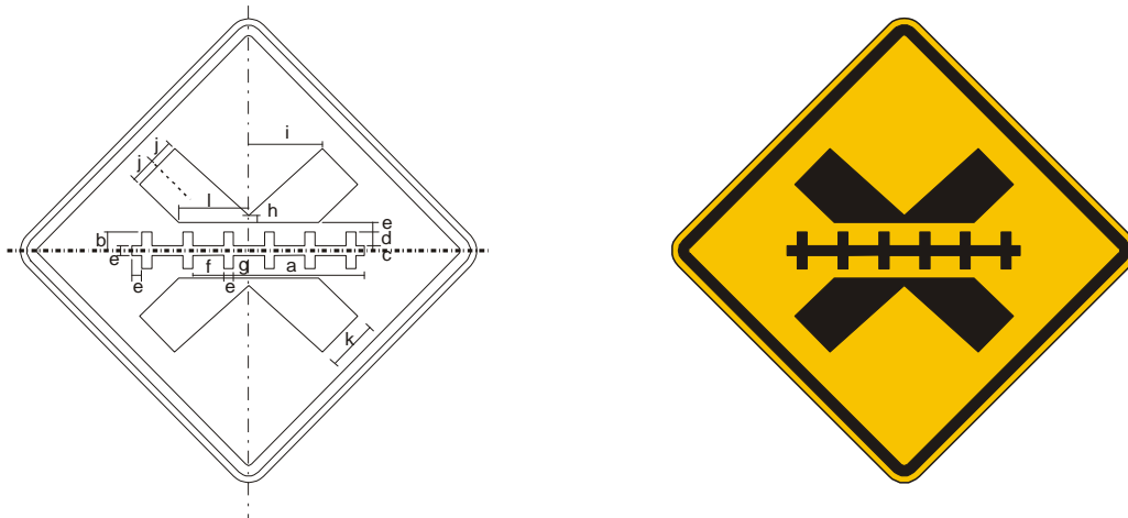
Figura A.111 – Placa A-39 – Passagem de nível sem barreira
