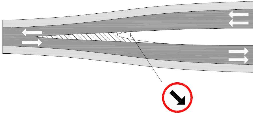
Figura 28 – Início de pista dupla
