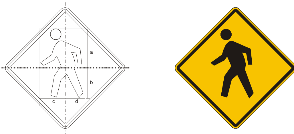
Figura A.102 – Placa A-32a – Trânsito de pedestres
