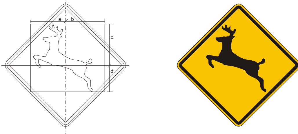
Figura A.108 – Placa A-36 – Animais selvagens
