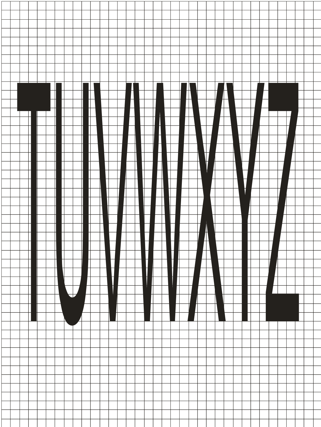
Figura A.152 – Letras T a Z – Para V \leq 60 km/h – Vias rurais
