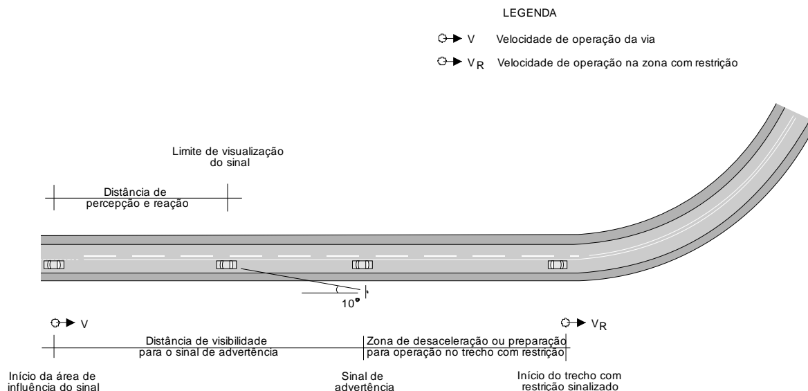
Figura 81 – Posicionamento longitudinal do sinal de advertência
