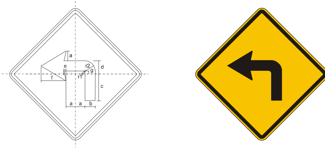
Figura A.55 – Placa A-1a – Curva acentuada à esquerda
