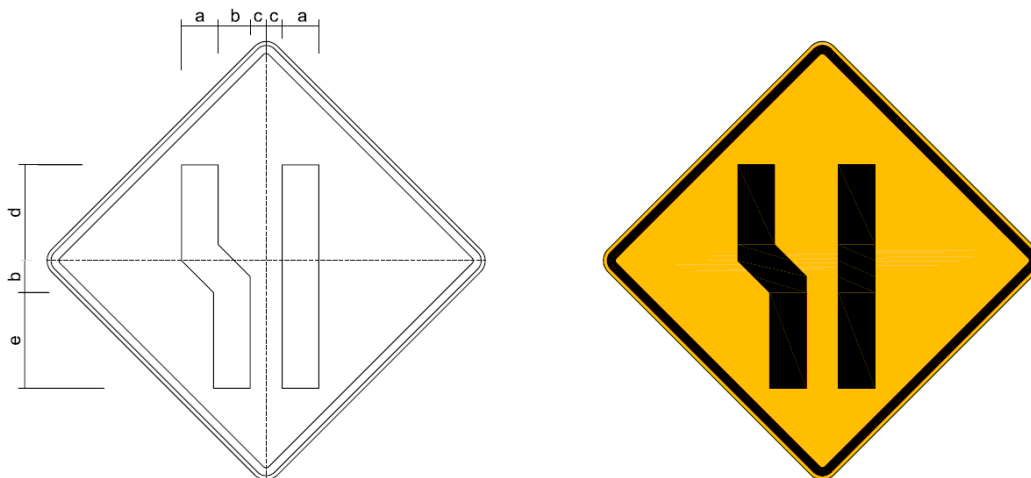
Figura A.88 – Placa A-21d – Alargamento de pista à esquerda
