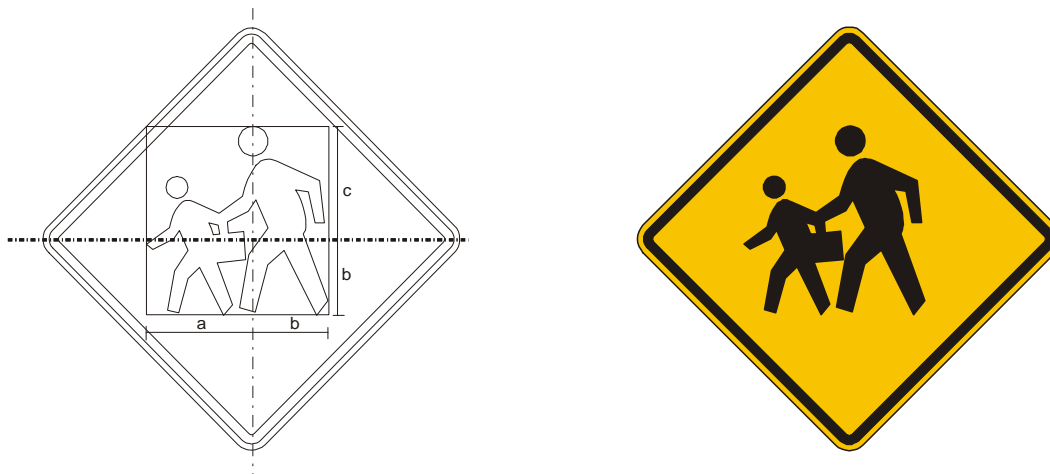
Figura A.104 – Placa A-33a – Área escolar
