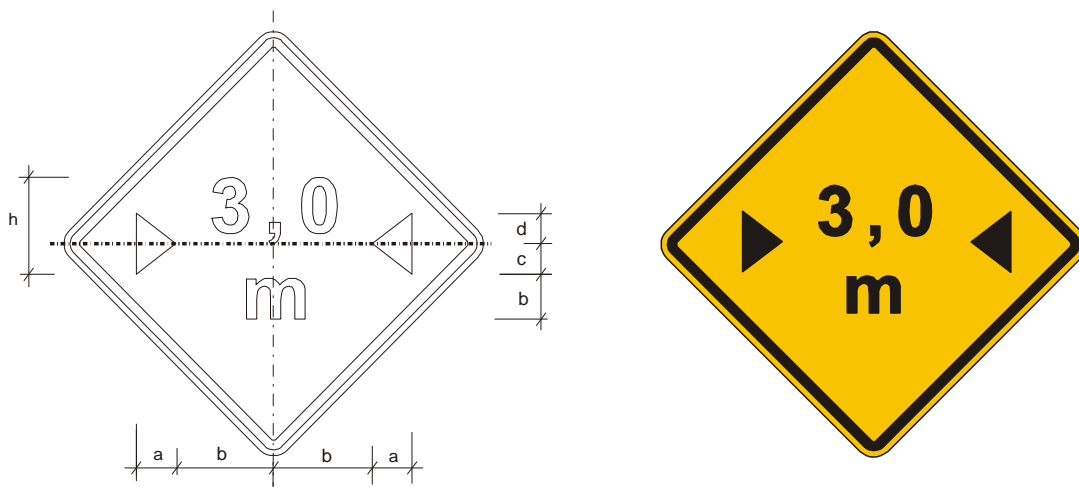
Figura A.110 – Placa A-38 – Largura limitada
