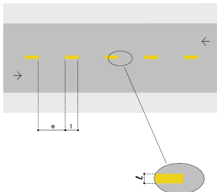
Figura 225 – Linha simples tracejada (LFO-2)
