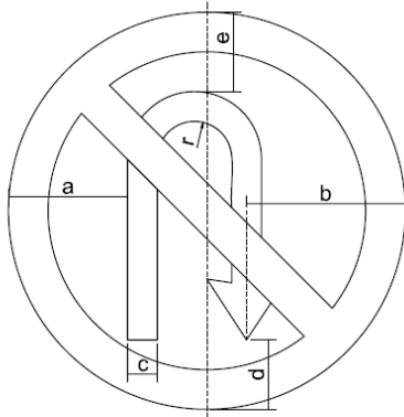
Figura A.9 – Placa R-5b – Proibido retornar à direita
