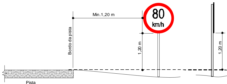
Figura 5 – Posicionamento dos sinais de regulamentação – Pista sem acostamento
