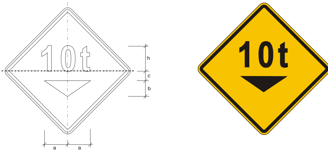
Figura A.119 – Placa A-46 – Peso bruto total limitado
