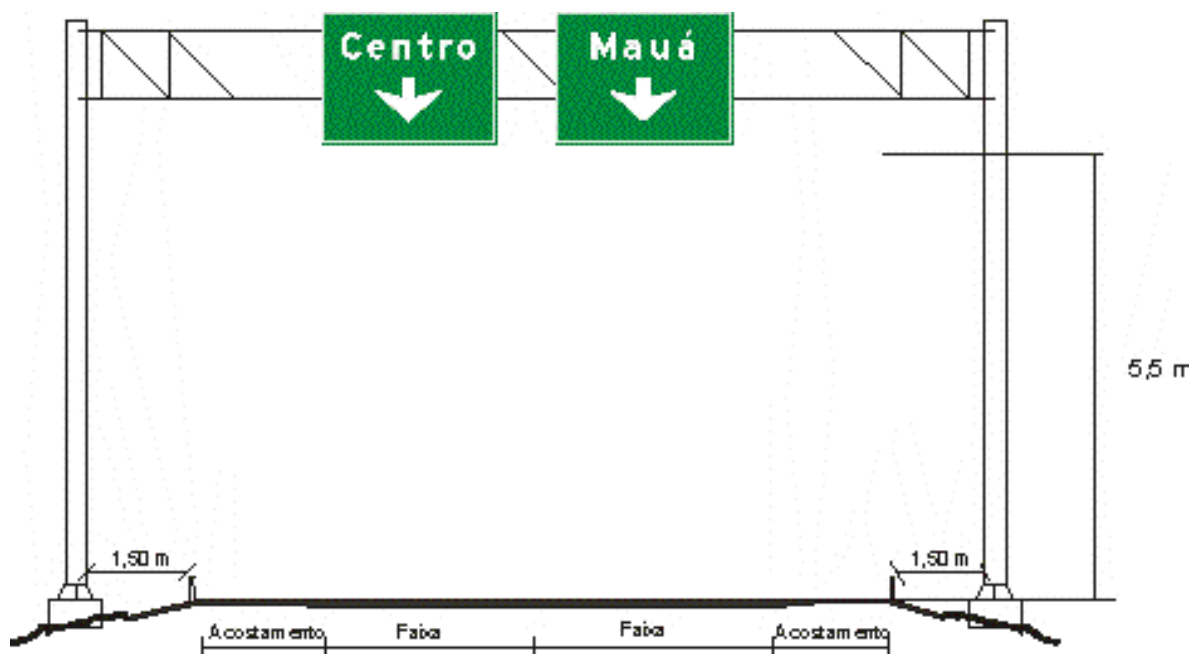
Figura 162 – Sinal em pórtico
