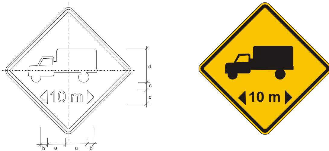
Figura A.121 – Placa A-48 – Comprimento limitado
