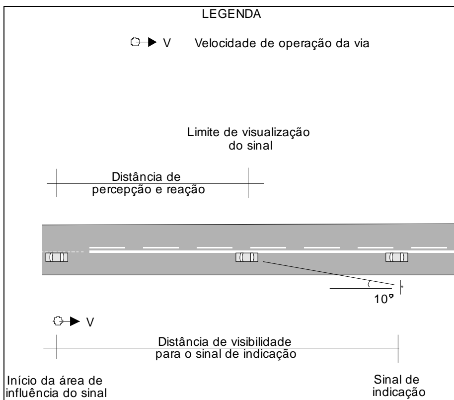
Figura 166 – Posicionamento longitudinal do sinal de indicação
