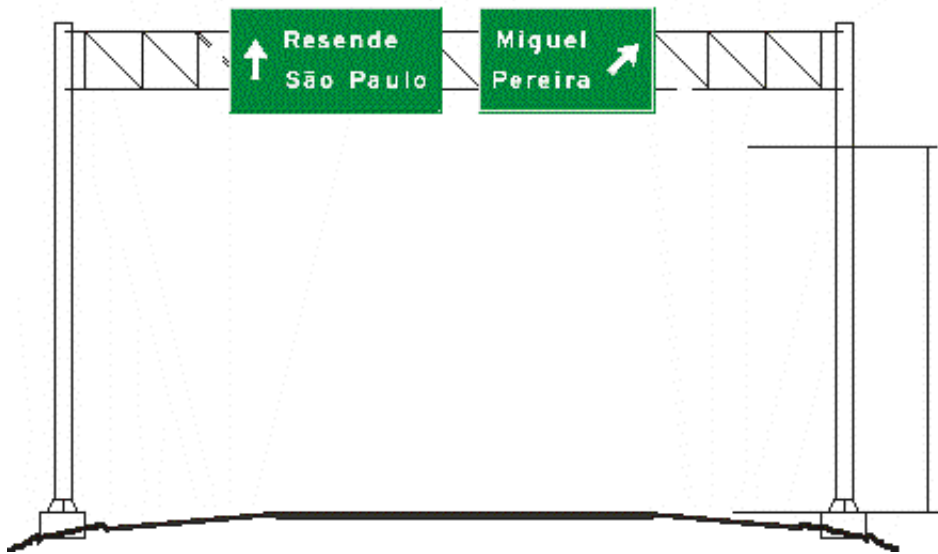
Figura 189 – Placa de pré – indicação em pórtico
