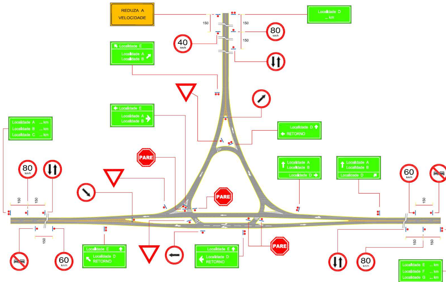
Figura 267 – Interseção em nível
