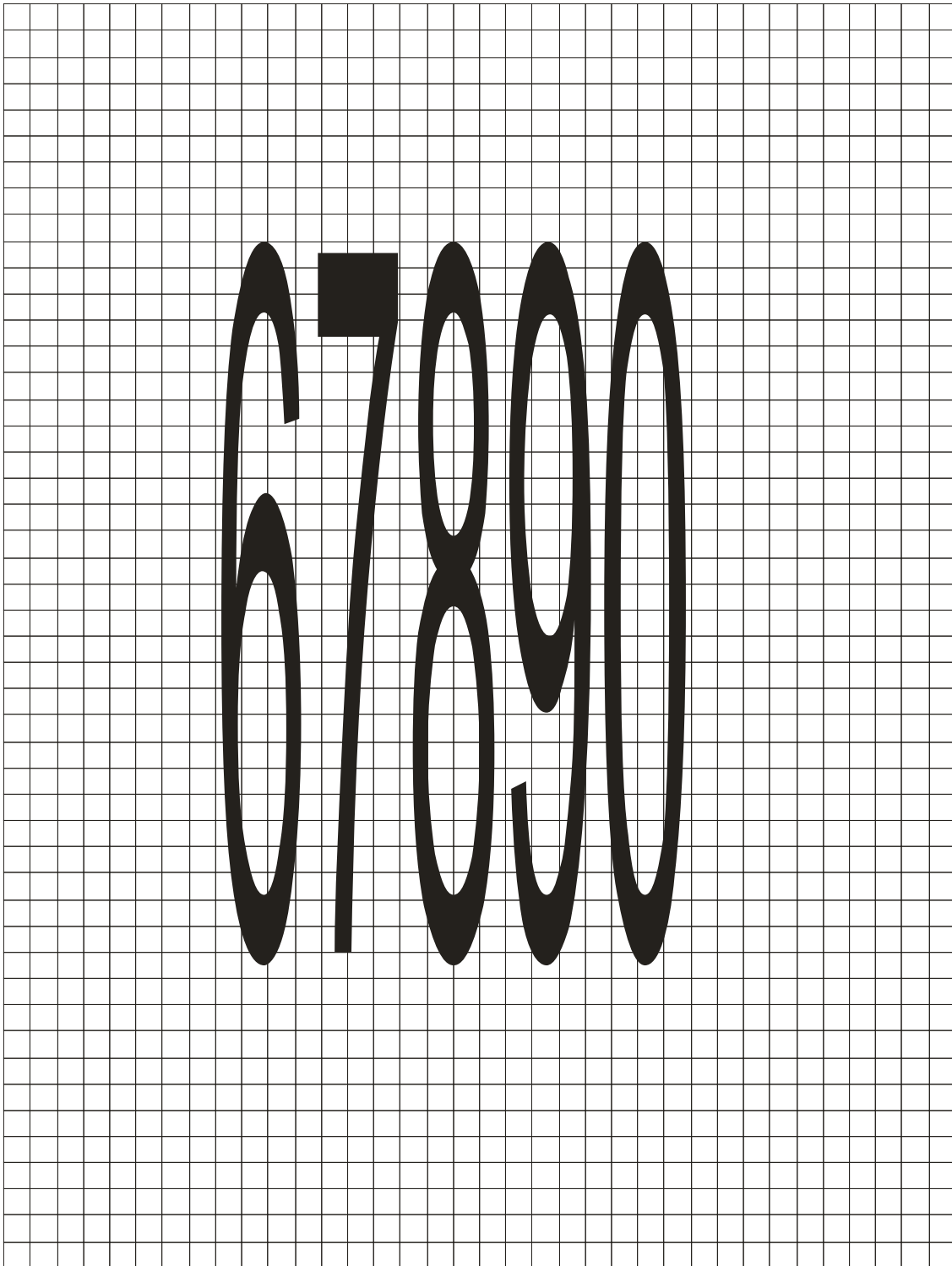
Figura A.154 – Números "6" a "0" – Para V \leq 60 km/h – Vias rurais
