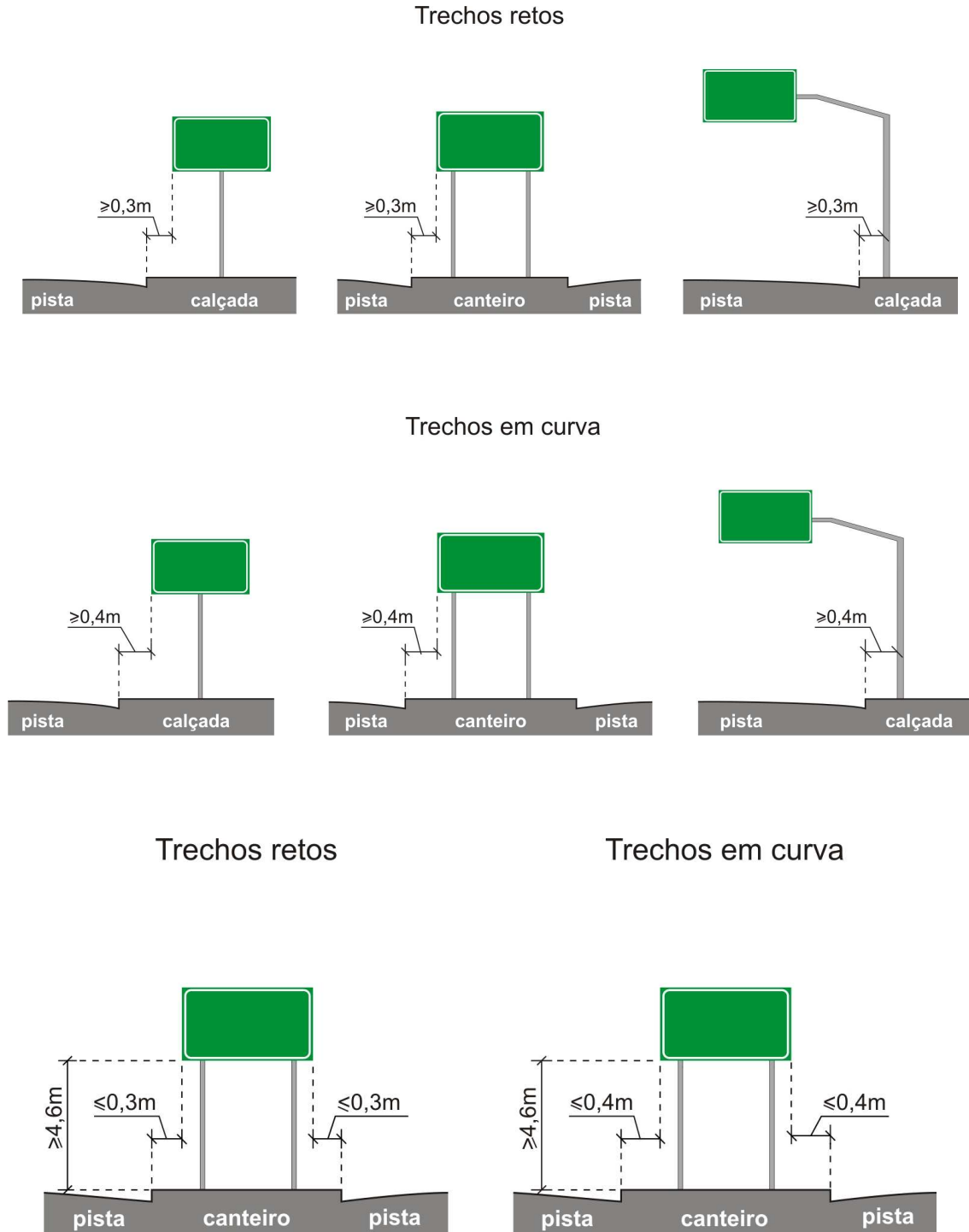
Figura 165 – Posicionamento na via – Vias urbanas
