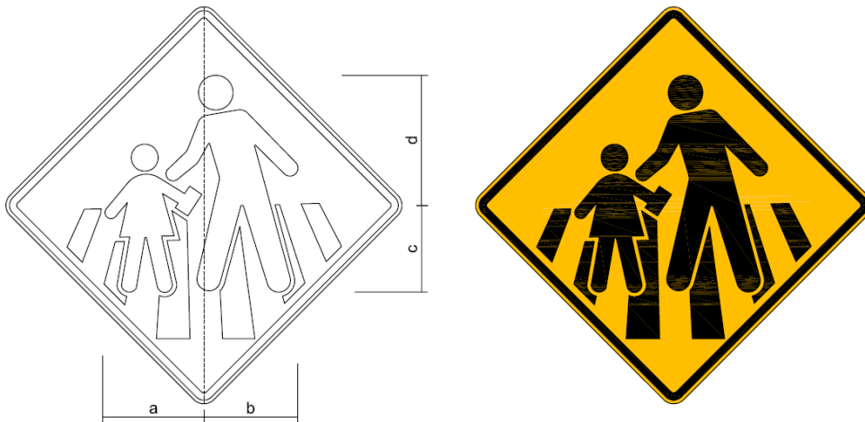
Figura A.105 – Placa A-33b – Passagem sinalizada de escolares
