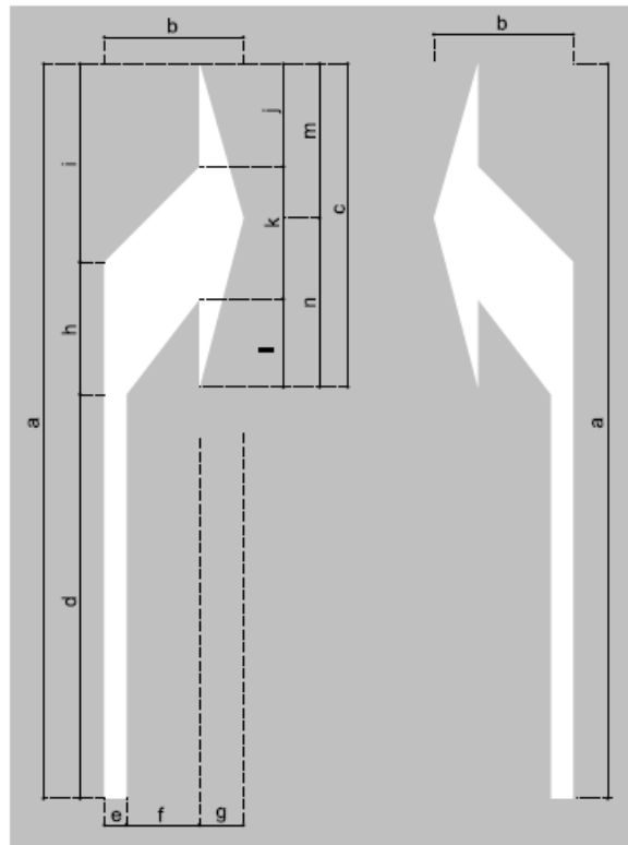
Figura 248 – Setas “vire à direita” e “vire à esquerda”
