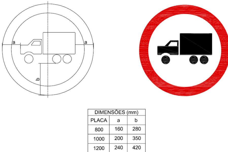
Figura A.52 – Placa R-39 – Circulação exclusiva de caminhão
