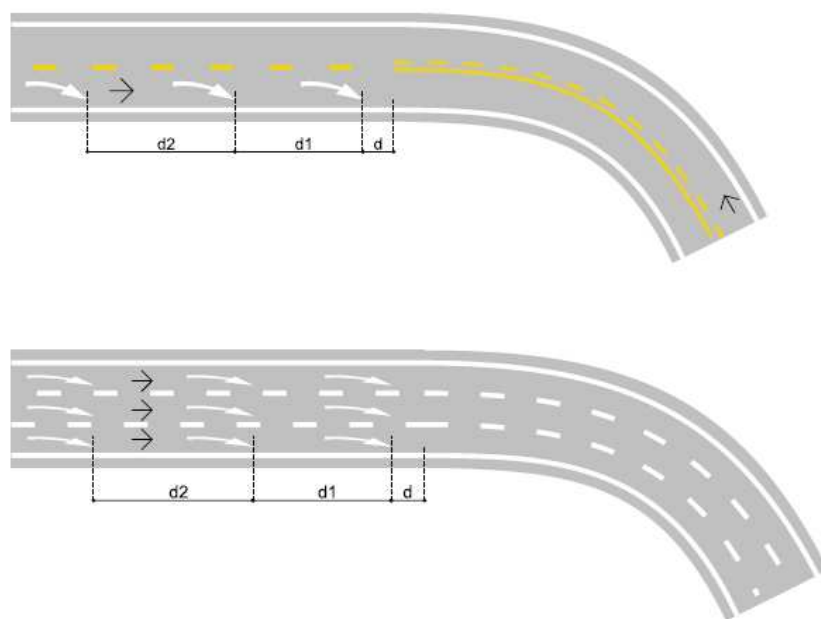
Figura 254 – Exemplos de uso de setas IMC
