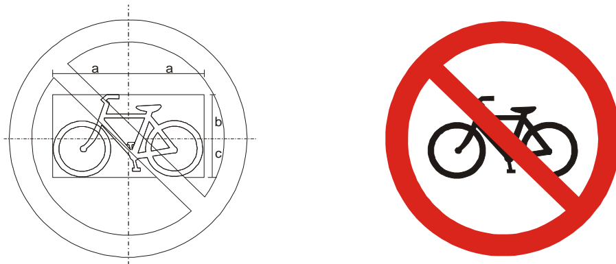
Figura A.19 – Placa R-12 – Proibido trânsito de bicicletas
