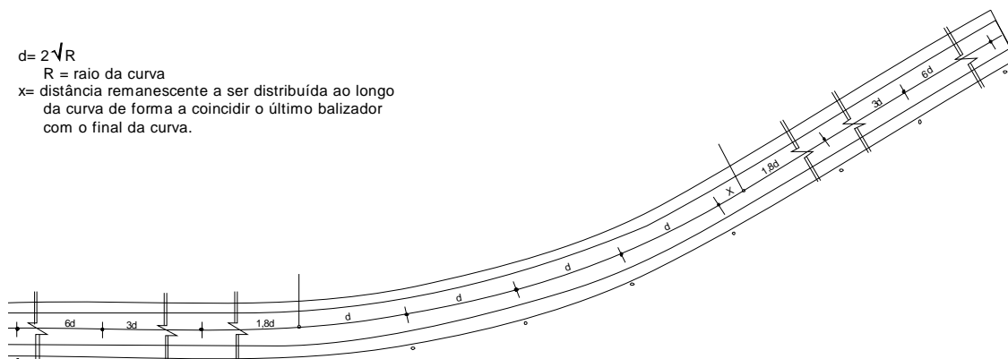
Figura 219 – Posicionamento dos balizadores em curva
