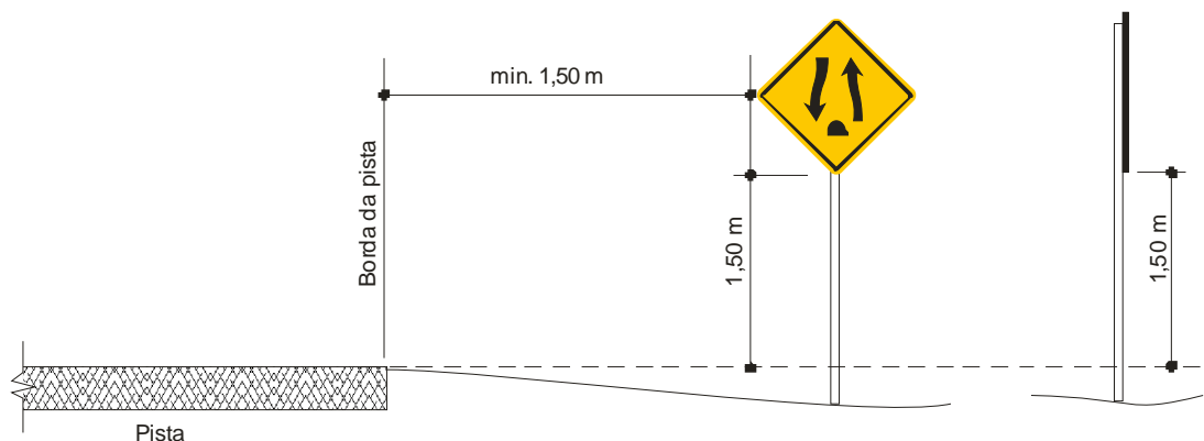
Figura 80 – Posicionamento transversal – Pista sem acostamento
