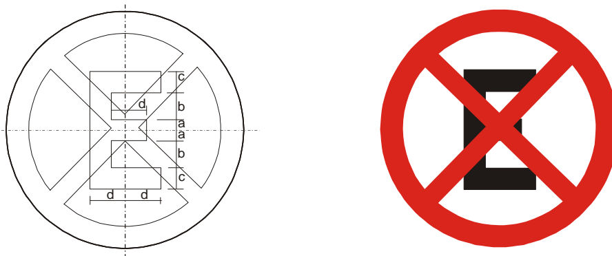
Figura A.12 – Placa R-6c – Proibido parar e estacionar
