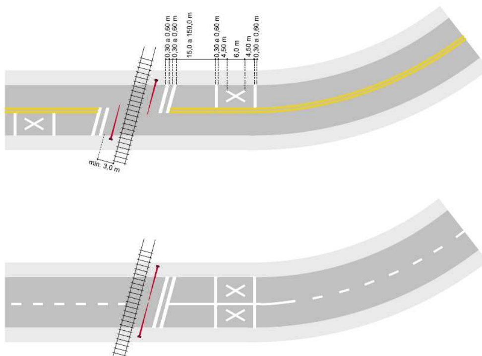
Figura 238 – Marcação de cruzamento rodoferroviário (MCF)
