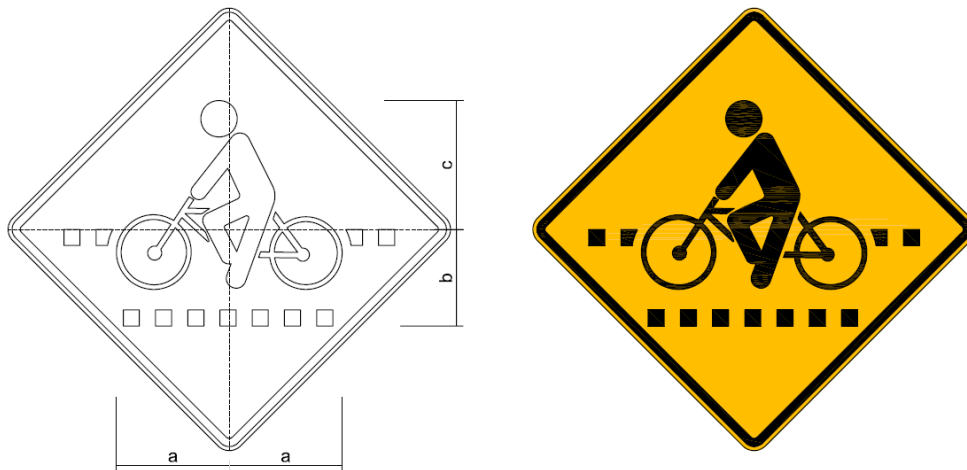
Figura A.99 – Placa A-30b – Passagem sinalizada de ciclistas
