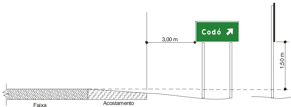
Figura 159 – Posicionamento transversal – Afastamento máximo
