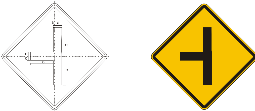
Figura A.66 – Placa A-7a – Via lateral à esquerda
