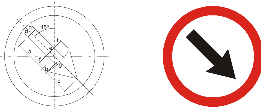
Figura A.32 – Placa R-24b – Passagem obrigatória
