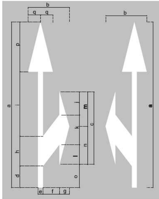
Figura 249 – Setas “siga em frente ou vire à direita” e “siga em frente ou vire à esquerda”
