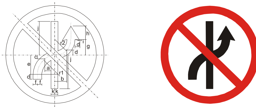
Figura A.14 – Placa R-8a – Proibido mudar de faixa ou pista de trânsito da esquerda para a direita
