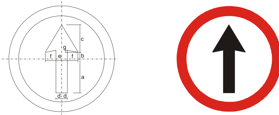
Figura A.37 – Placa R-26 – Siga em frente
