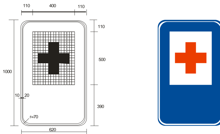
Figura A.128 – Placa I-7 – Pronto socorro
