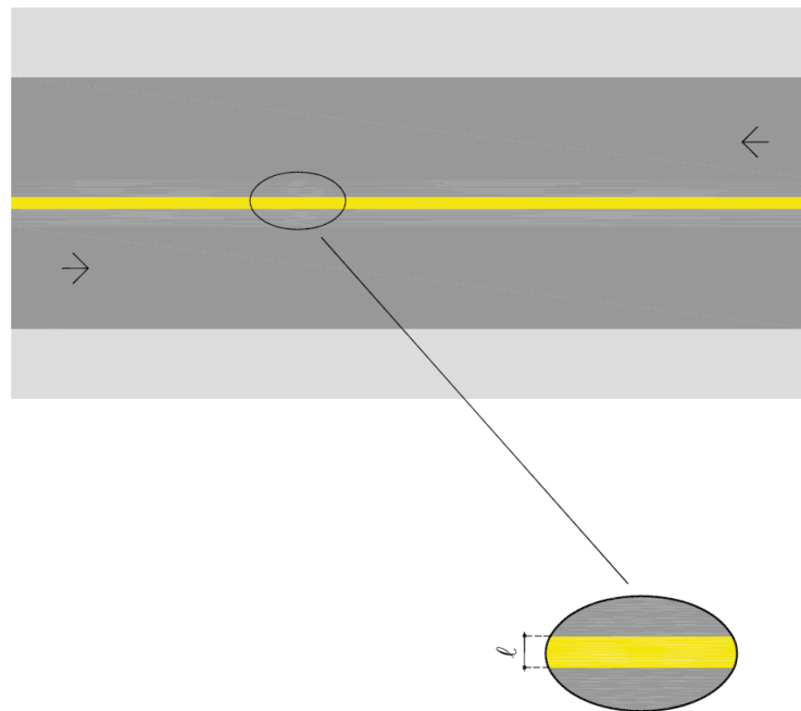
Figura 224 – Linha simples contínua (LFO-1)
