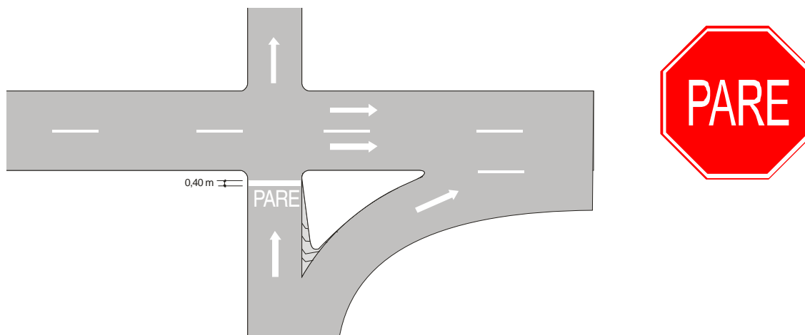
Figura 232 – Detalhe da linha de retenção de parada associada à placa PARE
