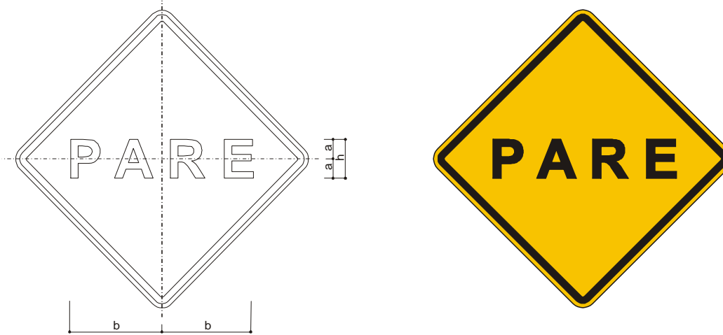
Figura A.78 – Placa A-15 – Parada obrigatória à frente
