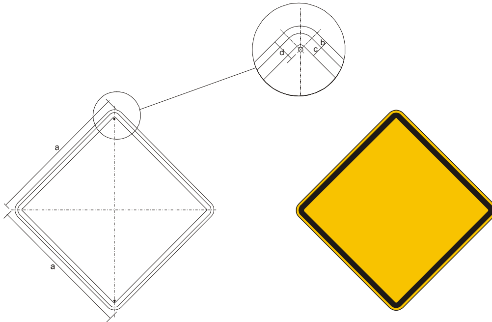
Figura A.54 – Desenho das orlas
