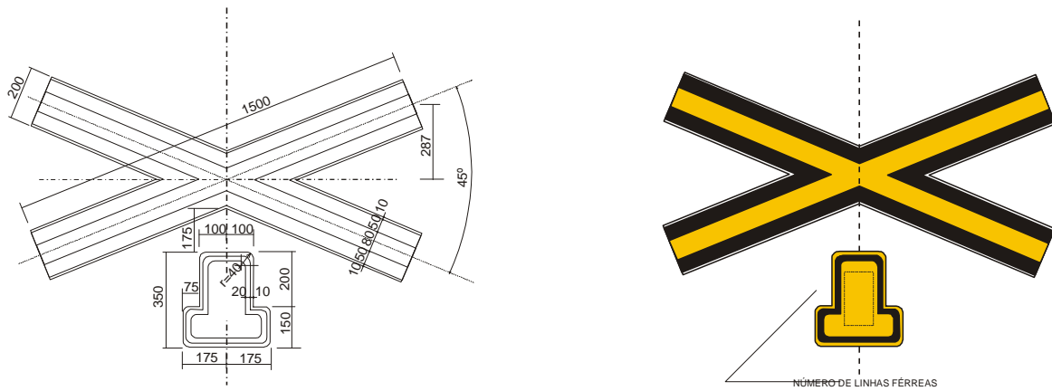
Figura A.113 – Placa A-41 – Cruz de santo andrè
