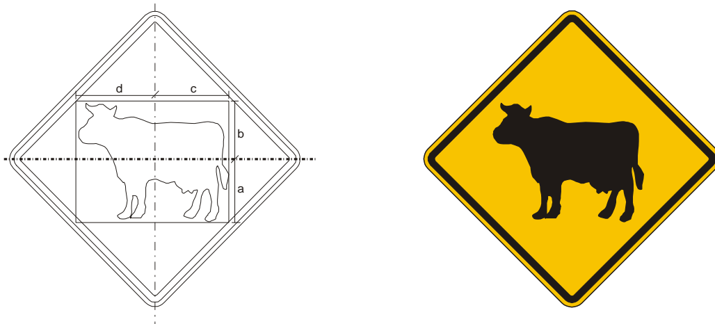
Figura A.107 – Placa A-35 – Animais
