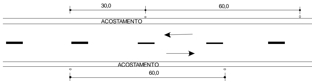
Figura 220 – Posicionamento dos balizadores em tangente
