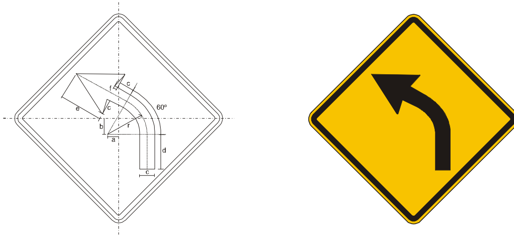
Figura A.57 – Placa A-2a – Curva à esquerda
