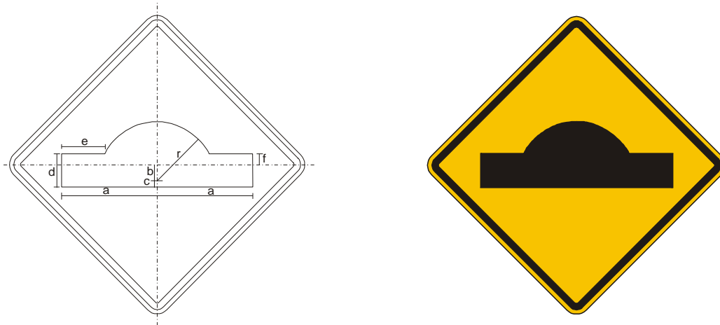
Figura A.81 – Placa A-18 – Saliência ou lombada
