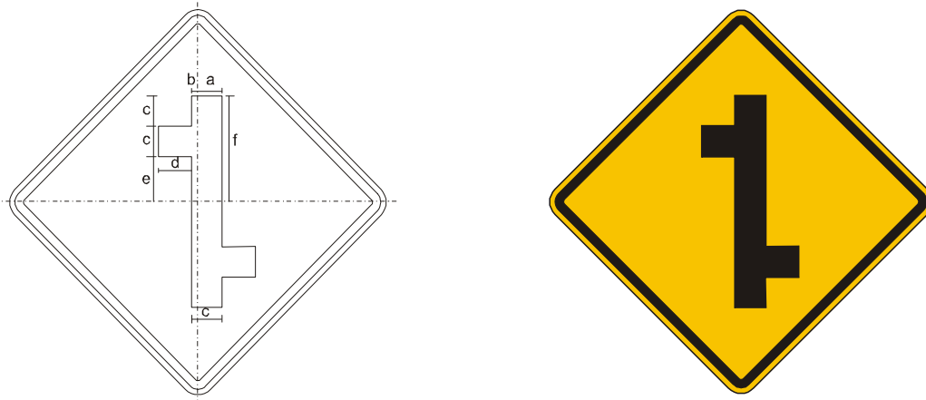
Figura A.73 – Placa A-11b – Junções sucessivas contrárias, primeira à direita
