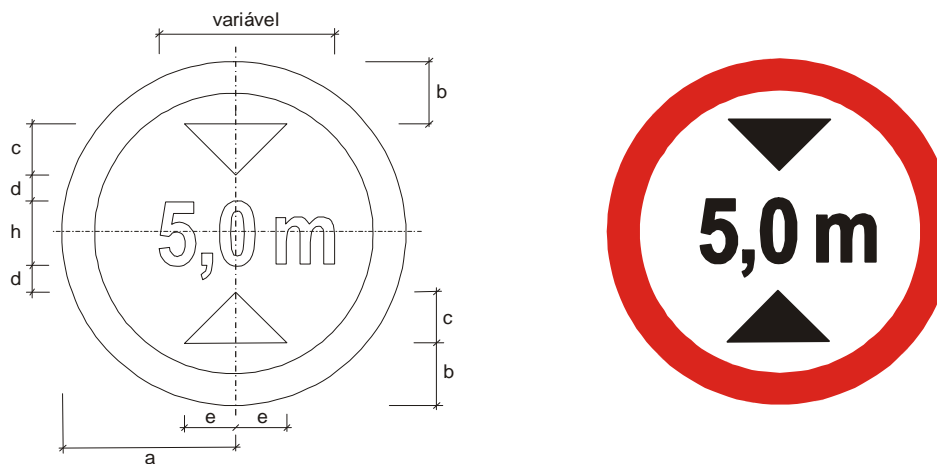
Figura A.22 – Placa R-15 – Altura máxima permitida
