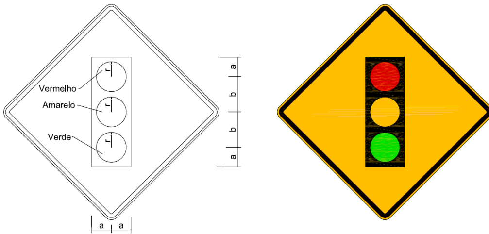
Figura A.77 – Placa A-14 – Semáforo à frente
