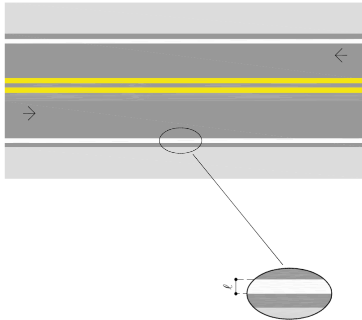
Figura 229 – Linha de borda (LBO)
