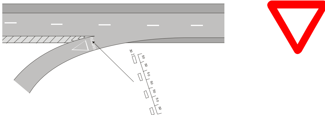
Figura 233 – Detalhe da linha “Dê a Preferência”
