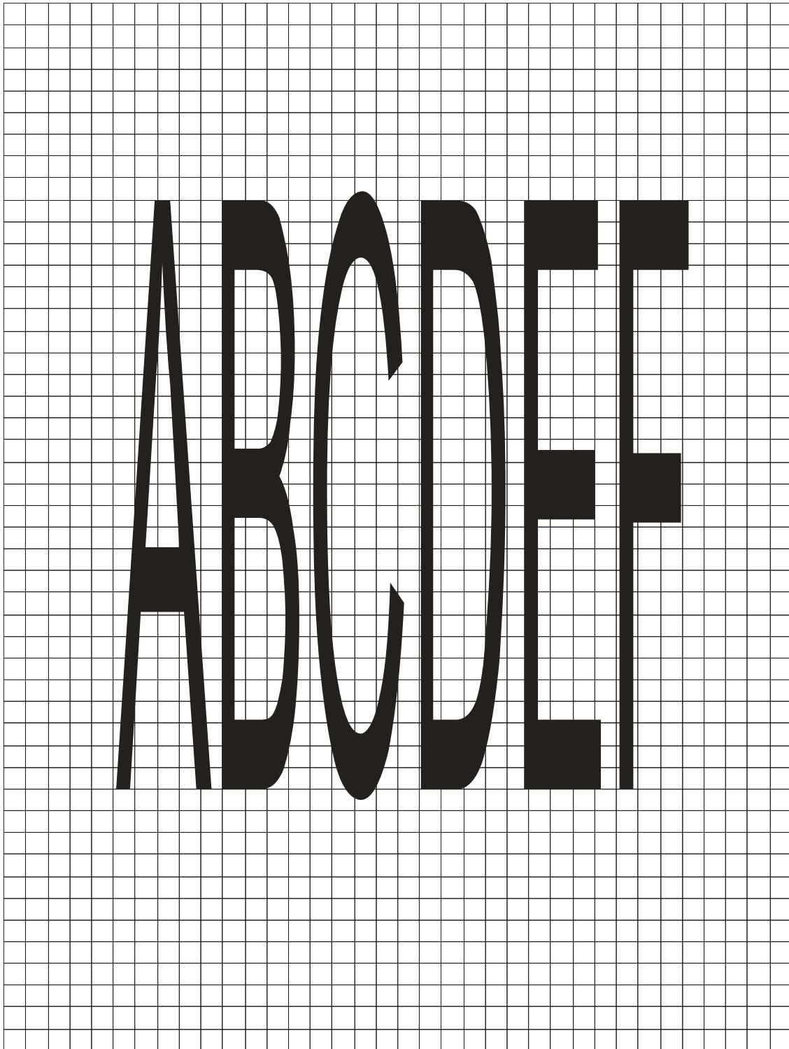
Figura A.149 – Letras A a F – Para V \leq 60 km/h – Vias / trechos rurais
