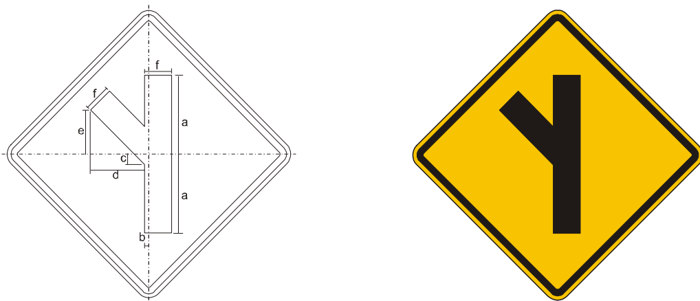
Figura A.70 – Placa A-10a – Entroncamento oblíquo à esquerda
