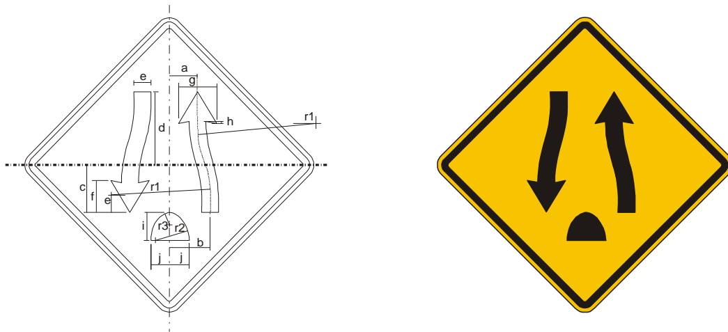
Figura A.115 – Placa A-42b – Fim de pista dupla
