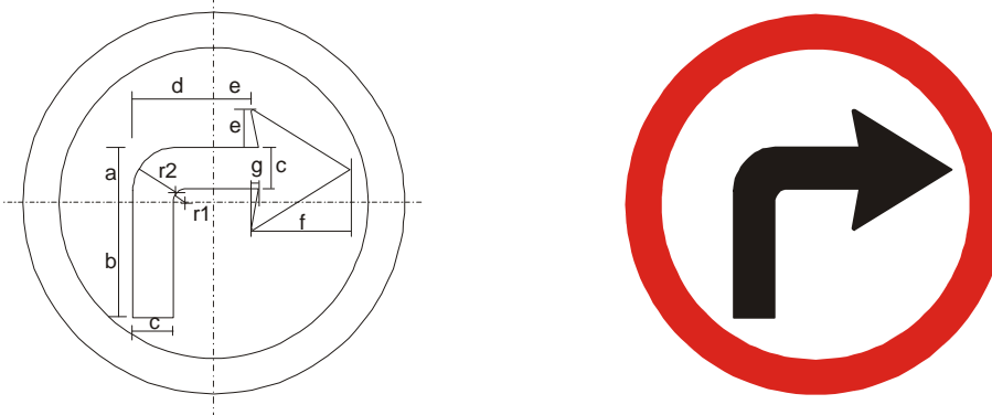
Figura A.34 – Placa R-25b – Vire à direita
