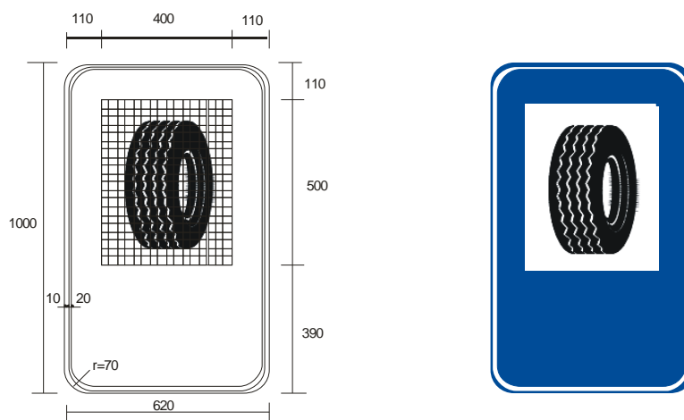
Figura A.134 – Placa I-13 – Borracheiro
