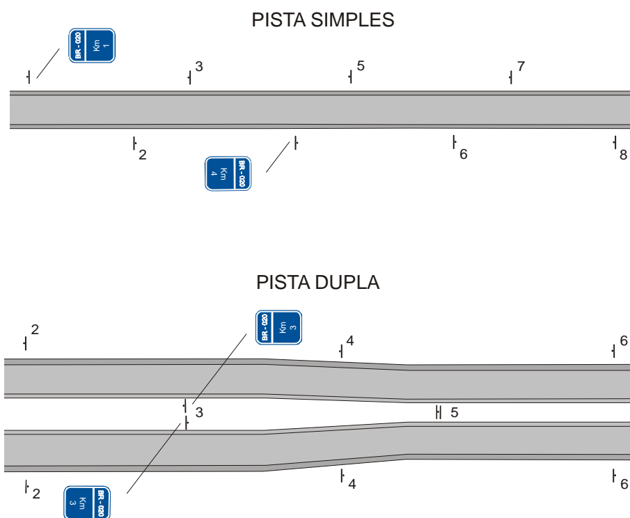
Figura 215 – Posicionamento longitudinal dos marcos
