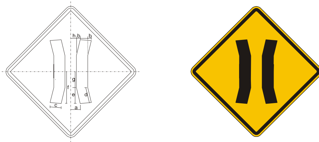
Figura A.90 – Placa A-22 – Ponte estreita
