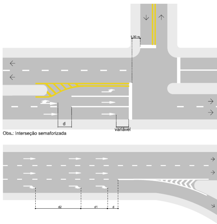
Figura 251 – Exemplos de uso de setas PEM
