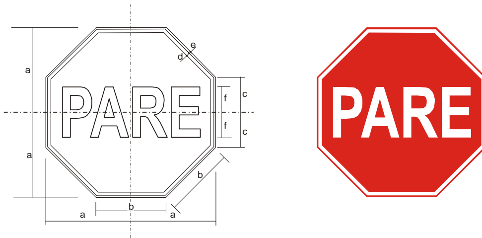
Figura A.3 – Placa R-1 – Parada obrigatória
