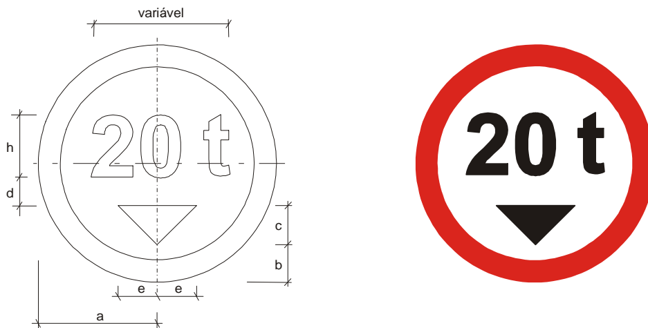
Figura A.21 – Placa R-14 – Peso bruto total máximo permitido
