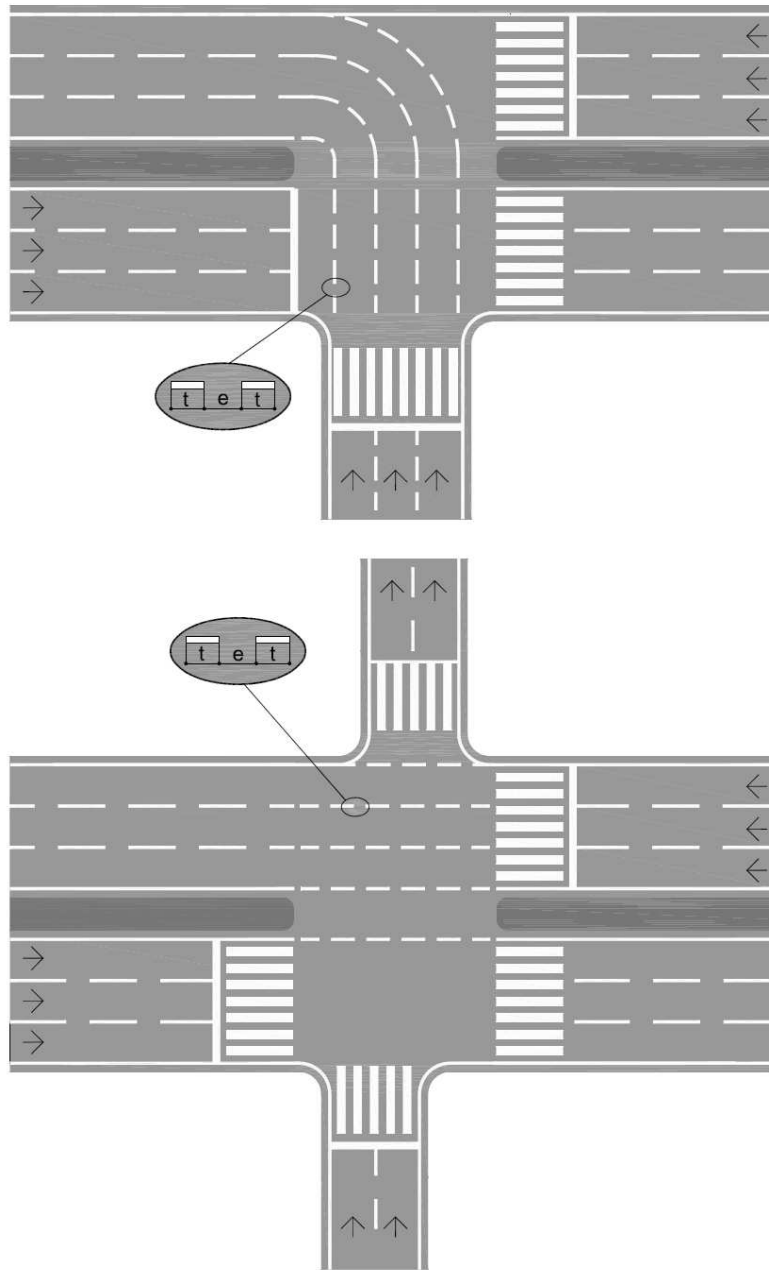
Figura 231 – Linha de continuidade (LCO)
