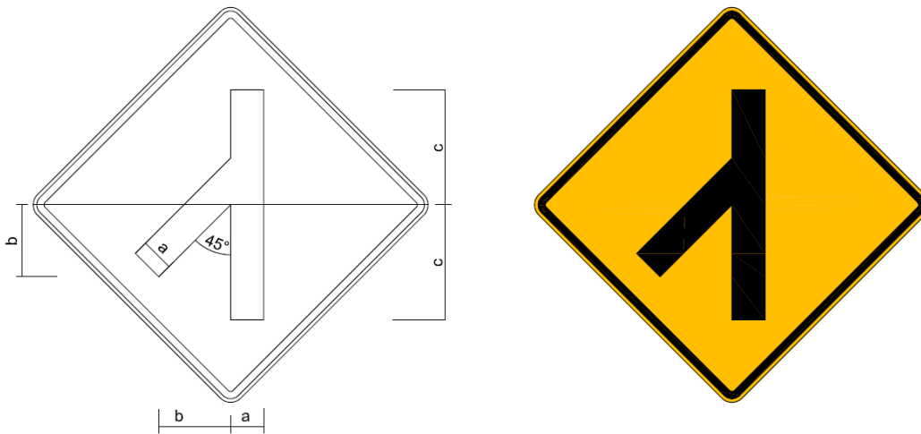
Figura A.75 – Placa A-13a – Confluência à esquerda
