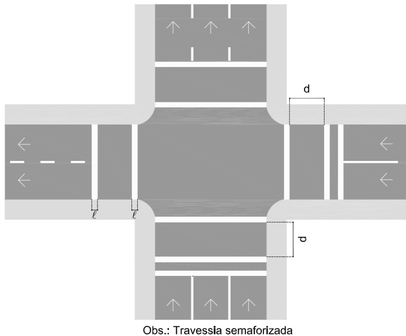
Figura 237 – Faixa de travessia – tipo paralela (FTP-2)
