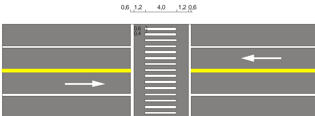
Figura 235 – Faixas de travessia de pedestres
