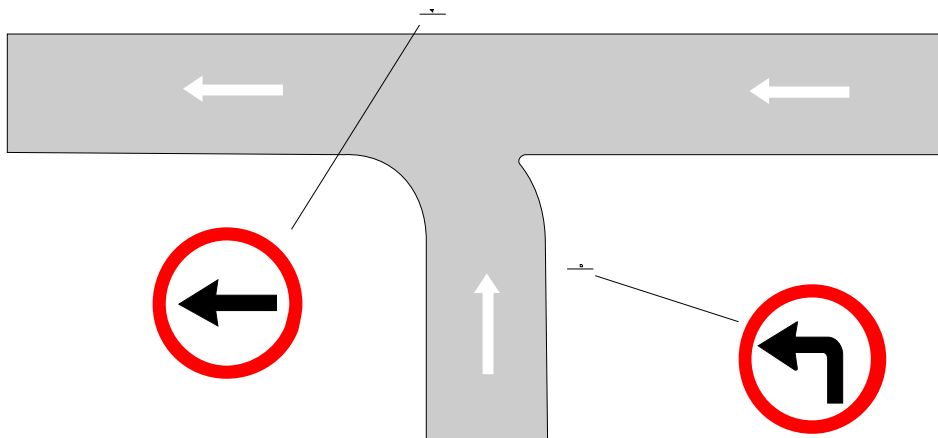
Figura 18 – Entroncamento com o sinal de sentido obrigatório – Movimento à esquerda
