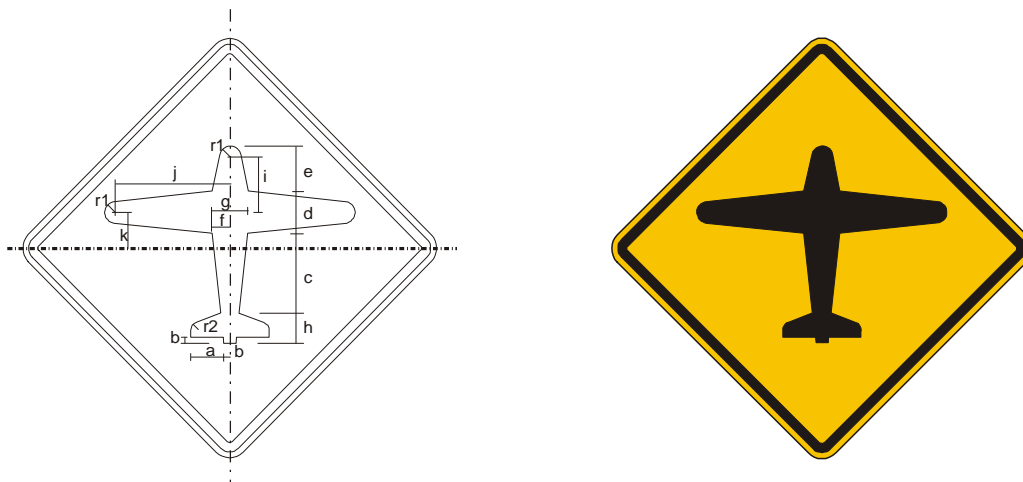
Figura A.116 – Placa A-43 – Aeroporto
