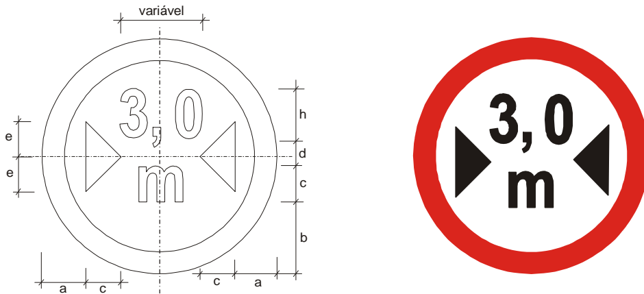
Figura A.23 – Placa R-16 – Largura máxima permitida
