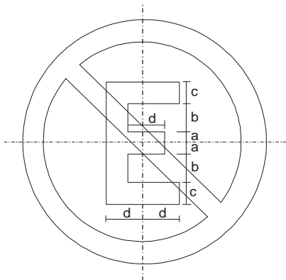
Figura A.10 – Placa R-6a – Proibido estacionar
