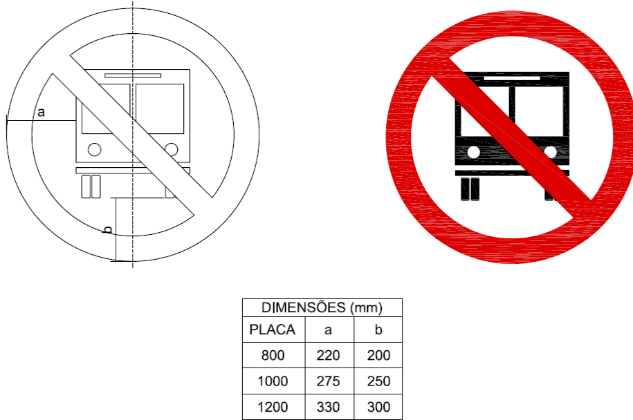
Figura A.51 – Placa R-38 – Proibido trânsito de ônibus
