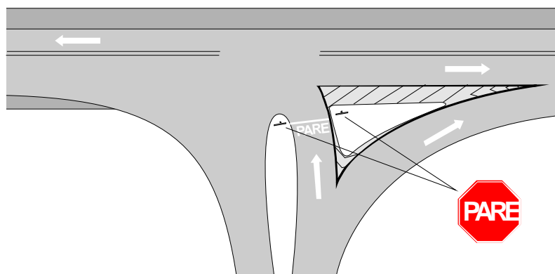
Figura 13 – Aproximação com ilha tipo gota e ilha triangular
