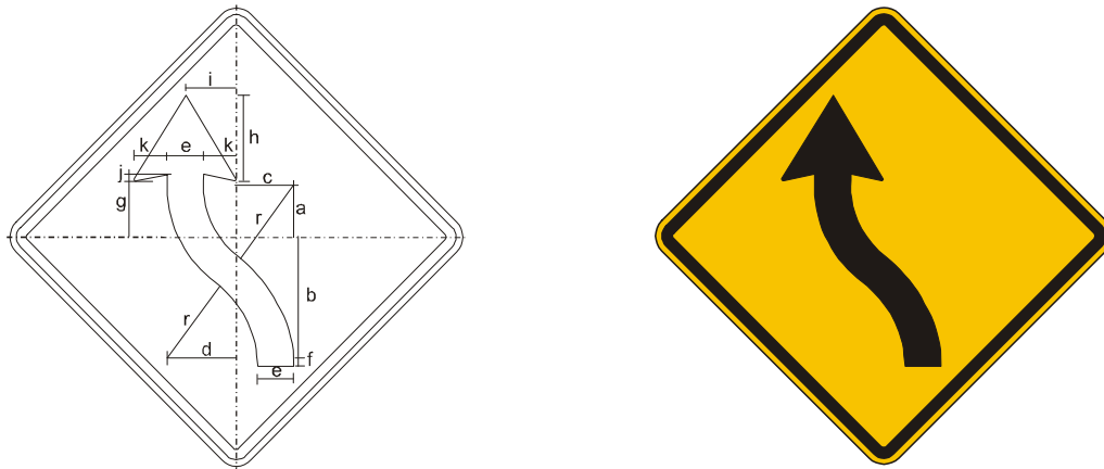
Figura A.63 – Placa A-5a – Curva em “S” à esquerda
