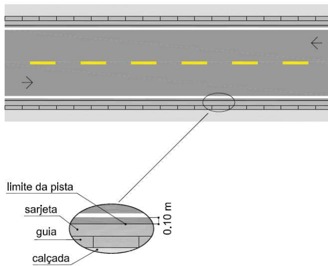
Figura 230 – Linha de borda de pista
