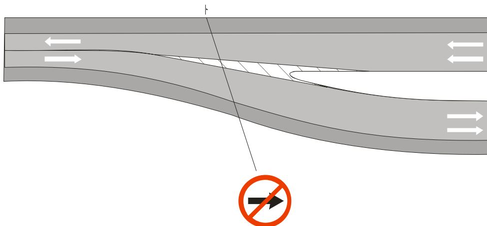
Figura 57 – Transição pista dupla – pista simples
