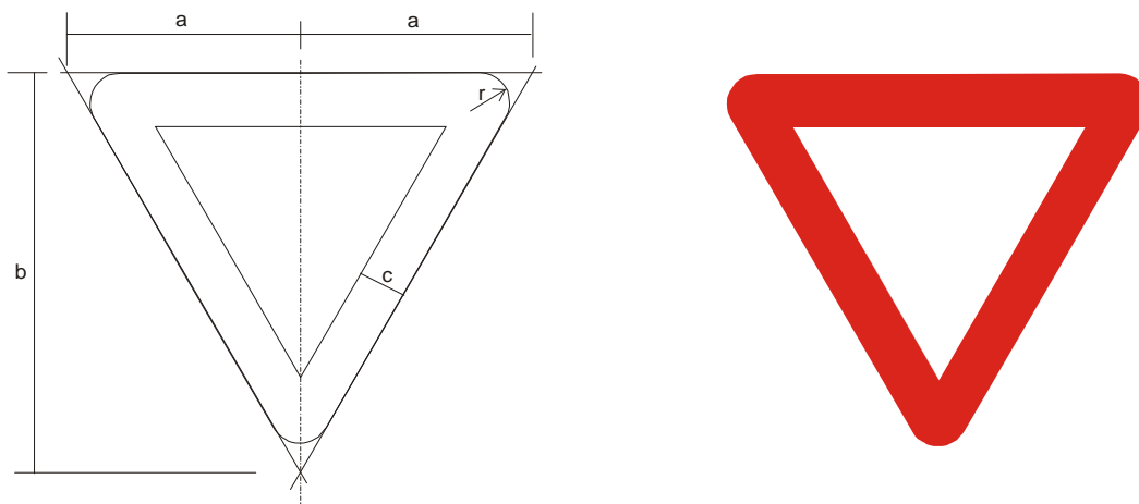
Figura A.4 – Placa R-2 – Dê a Preferência
