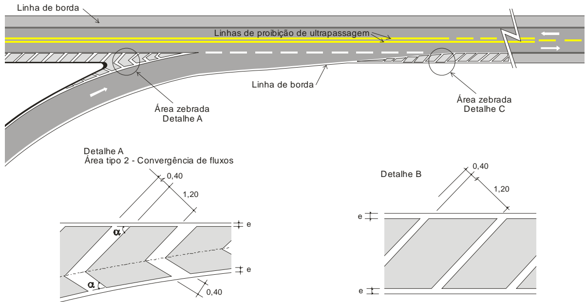
Figura 240 – Exemplo de sinalização horizontal para entrada de ramo de uma faixa
