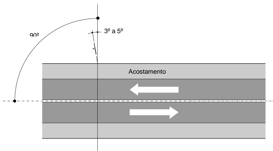
Figura 160 – Posicionamento transversal – Inflexão em relação à via
