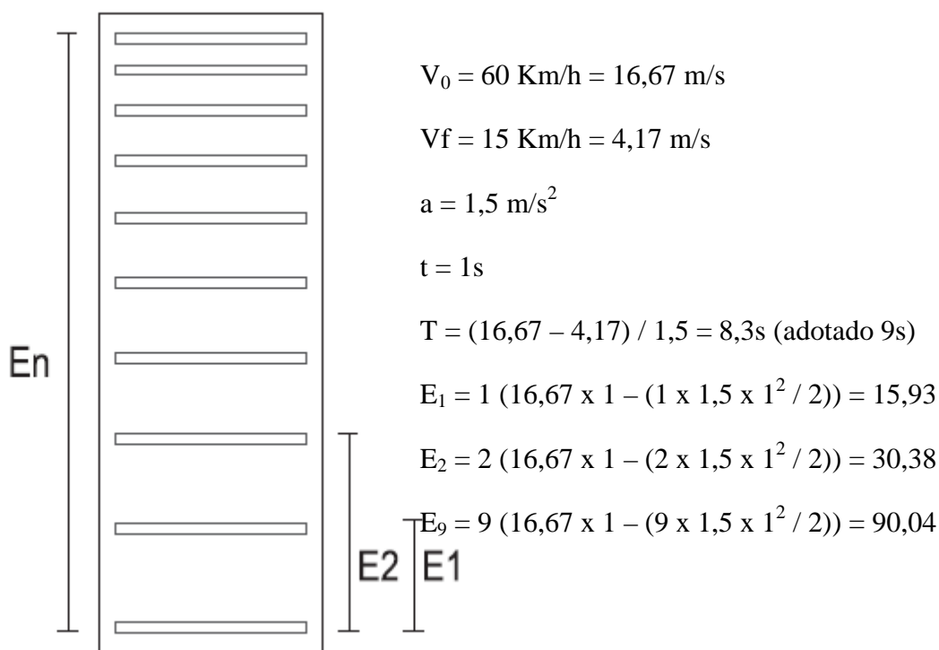
Figura 234 – Linhas de estímulo à redução de velocidade
