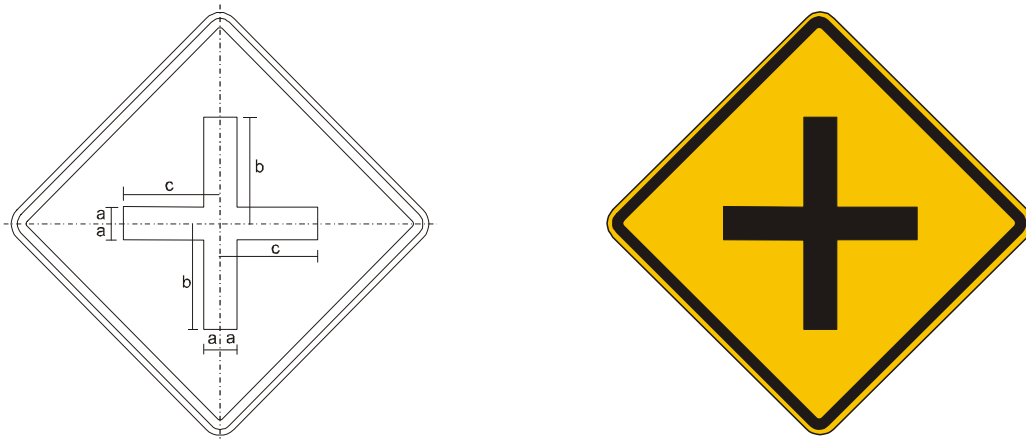
Figura A.65 – Placa A-6 – Cruzamento de vias
