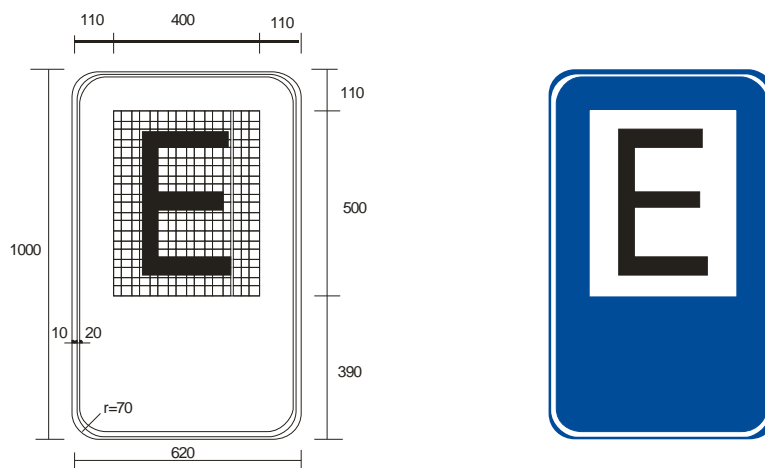
Figura A.131 – Placa I-10 – Área de estacionamento
