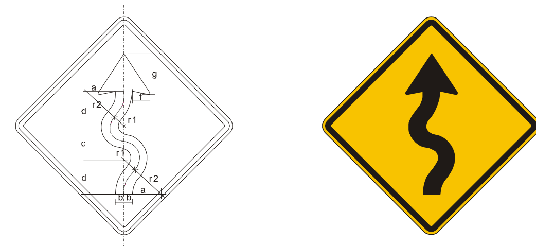
Figura A.60 – Placa A-3b – Pista sinuosa à direita
