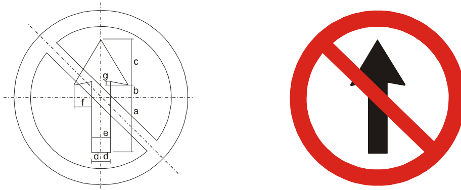
Figura A.5 – Placa R-3 – Sentido proibido
