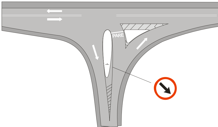
Figura 29 – Interseção tipo gota
