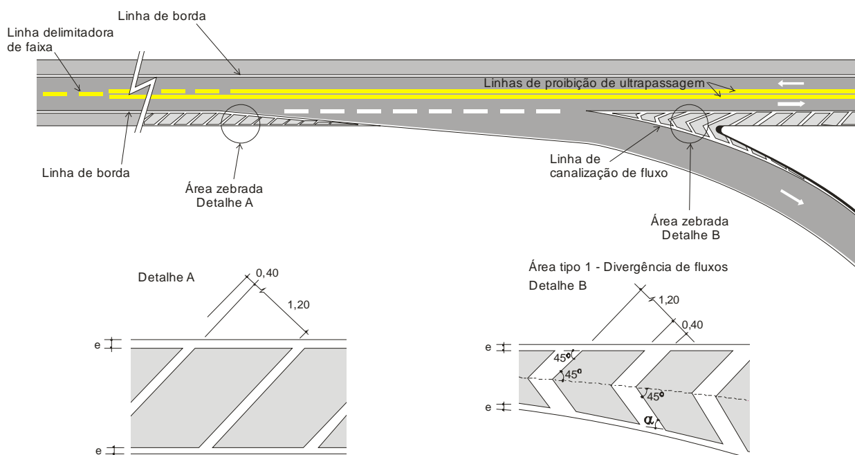
Figura 239 – Exemplo de sinalização horizontal para saída de ramo de uma faixa
