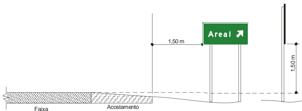
Figura 158 – Posicionamento transversal – Recomendação padrão
