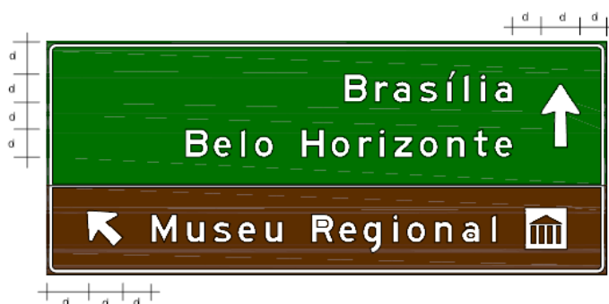
Figura 173 – Espaçamentos entre elementos – Mensagens com setas e pictograma
