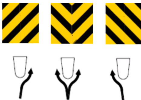
Figura 217 – Marcadores de obstáculos
