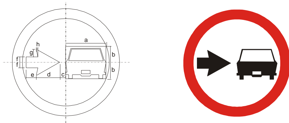
Figura A.30 – Placa R-23 – Conserve-se à direita
