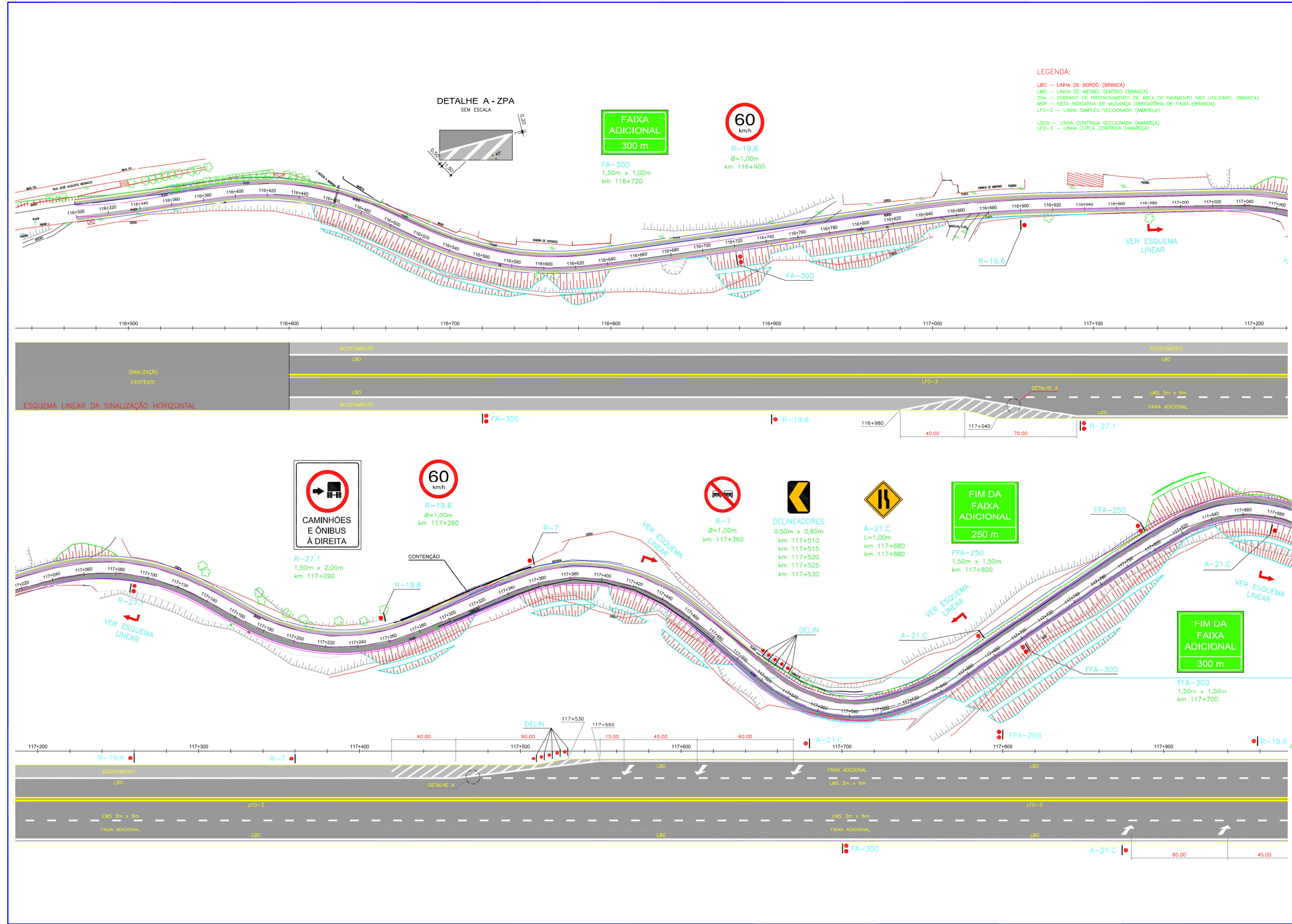
Figura 264 – Modelo de projeto de sinalização
