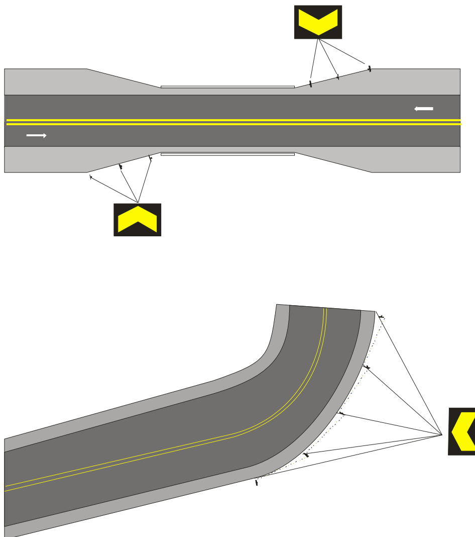
Figura 218 – Delineador e exemplos de utilização
