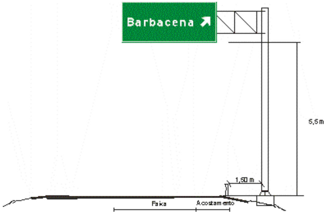
Figura 163 – Sinal em semipórtico
