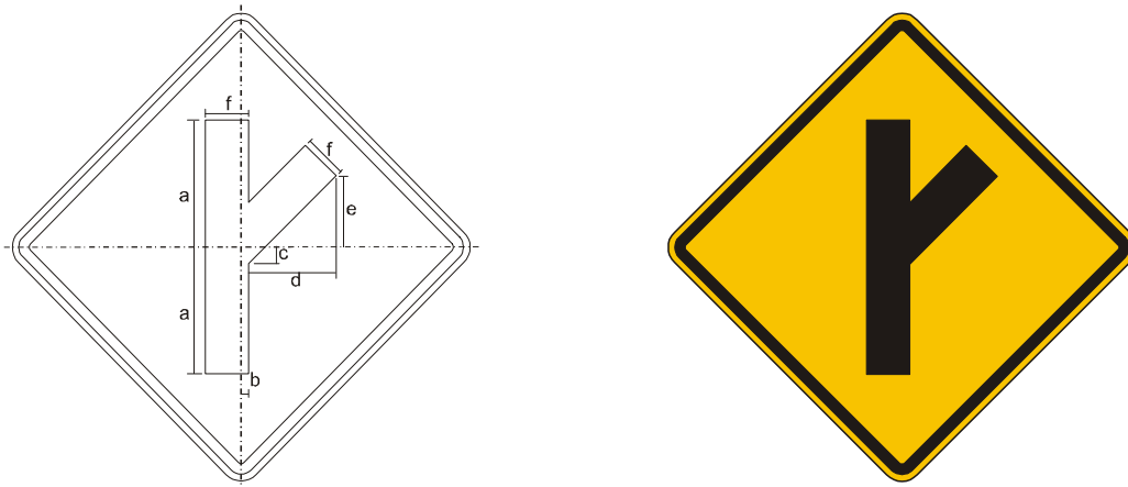
Figura A.71 – Placa A-10b – Entroncamento oblíquo à direita
