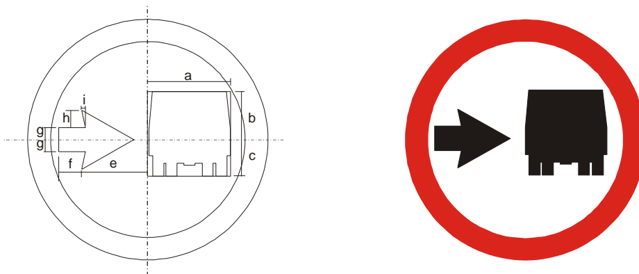
Figura A.38 – Placa R-27 – Ônibus, caminhões e veículos de grande porte mantenham-se à direita
