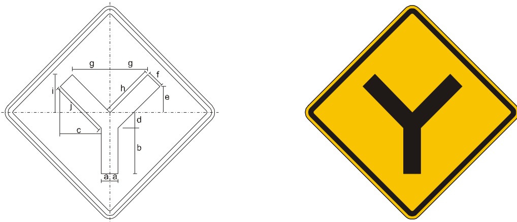
Figura A.69 – Placa A-9 – Bifurcação em “Y”
