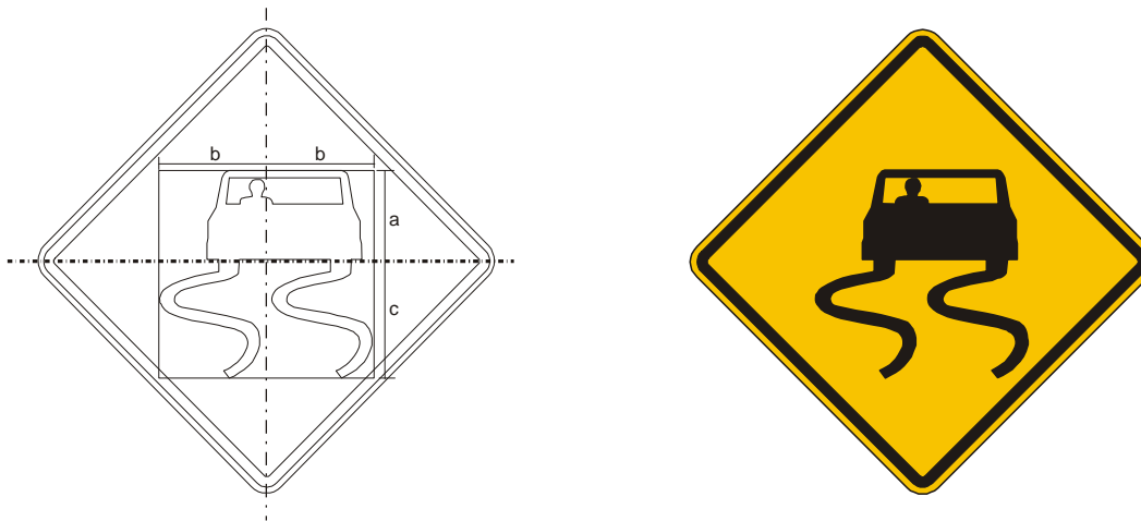
Figura A.96 – Placa A-28 – Pista escorregadia
