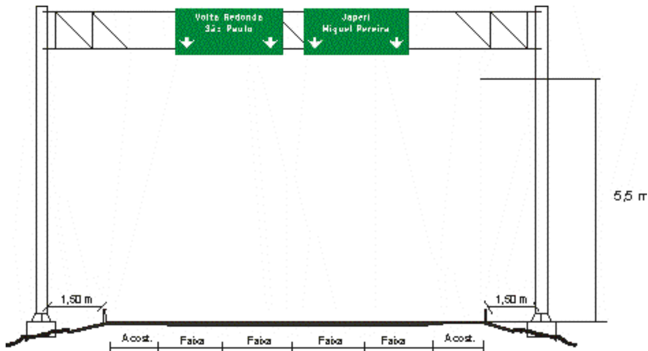
Figura 194 – Placas em pórticos sinalizando as faixas
