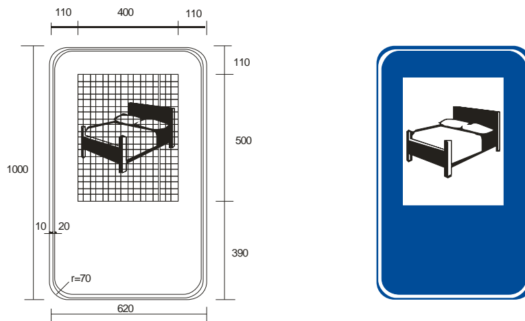
Figura A.127 – Placa I-6 – Hotel
