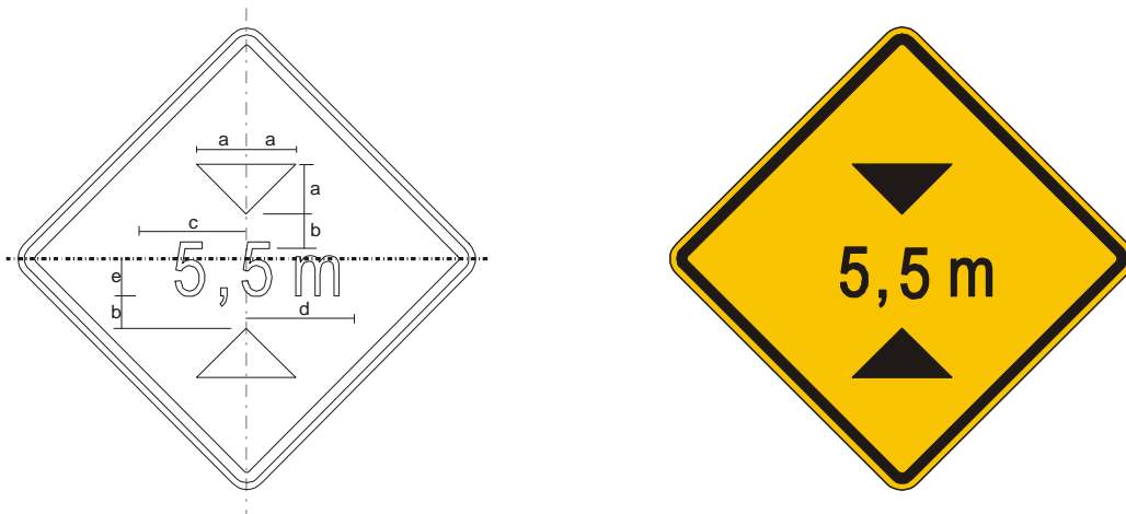
Figura A.109 – Placa A-37 – Altura limitada
