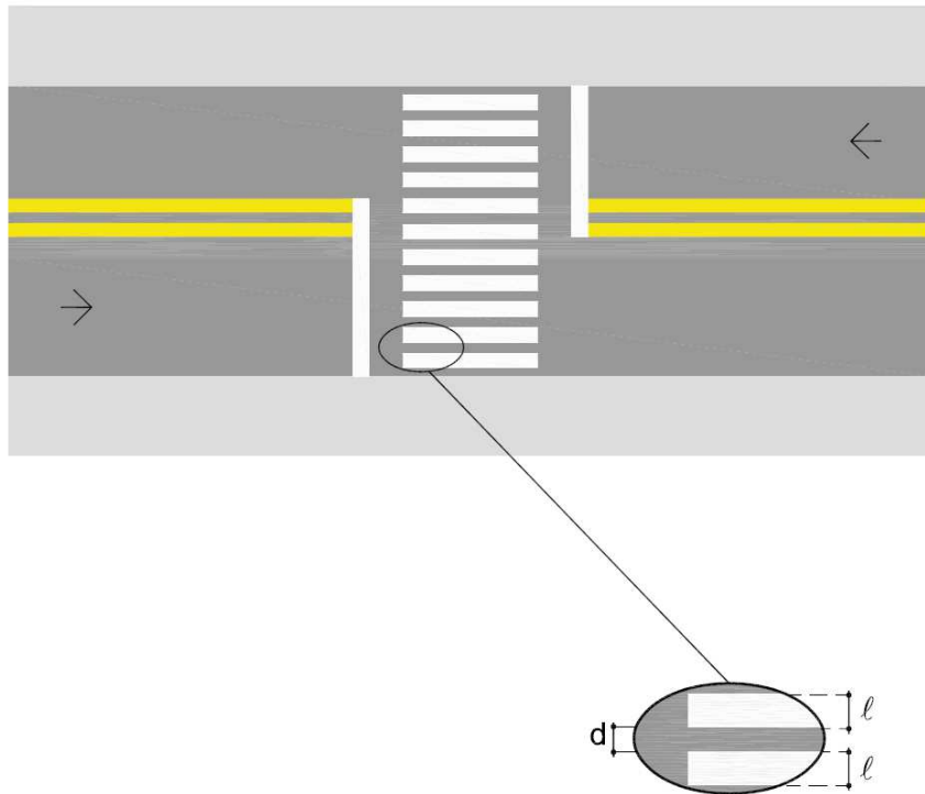
Figura 237 – Faixa de travessia – tipo paralela (FTP-2)
