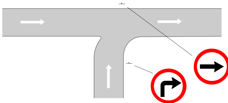
Figura 19 – Entroncamento com o sinal de sentido obrigatório – Movimento à direita
