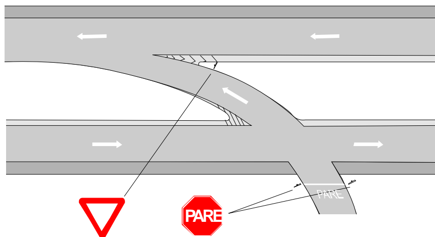
Figura 16 – Conversão à esquerda em pista dupla com canteiro maior que 10 m
