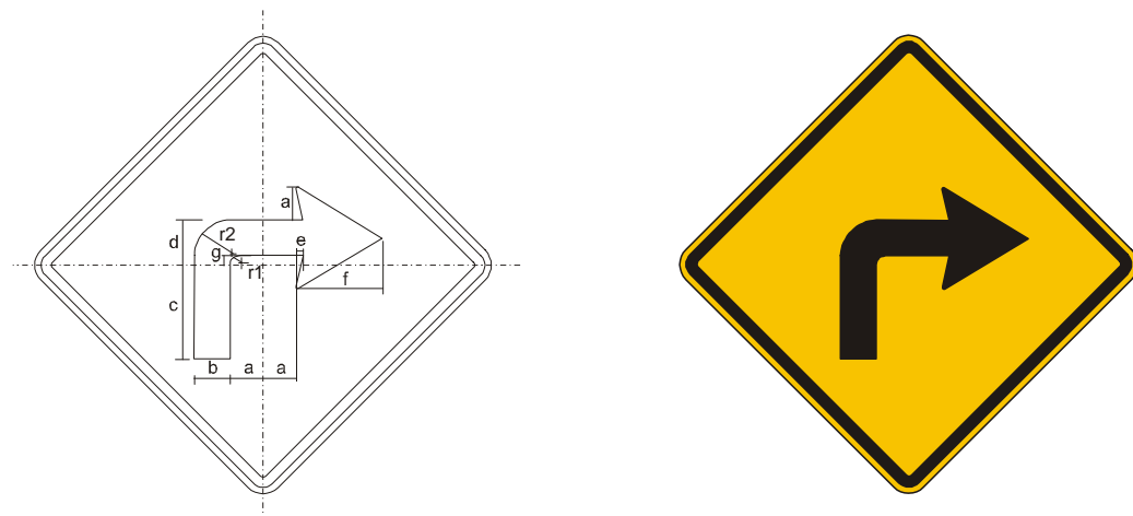
Figura A.56 – Placa A-1b – Curva acentuada à direita
