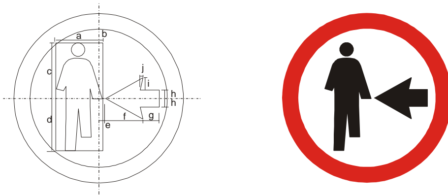
Figura A.41 – Placa R-30 – Pedestre, ande pela esquerda
