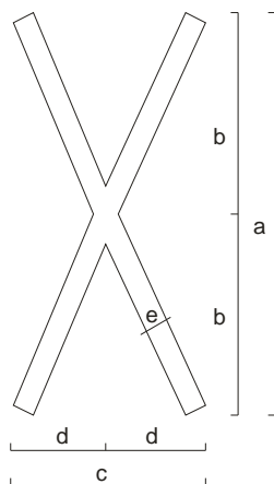
Figura 256 – Símbolo da Cruz de Santo André
