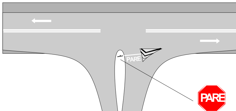
Figura 12 – Aproximação com ilha tipo gota sem ilha triangular
