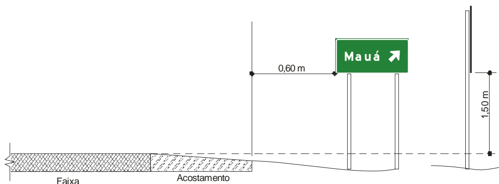
Figura 161 – Posicionamento transversal – Casos excepcionais
