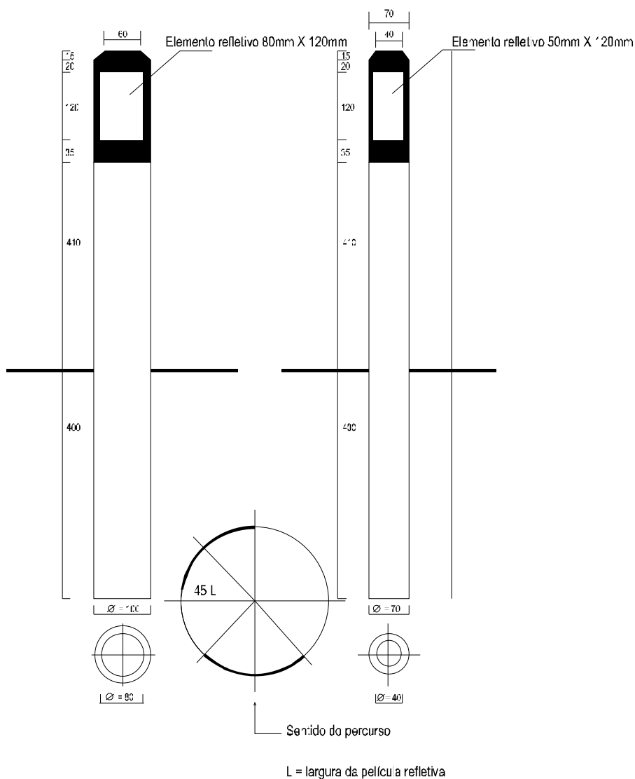
Figura 221 – Balizadores-tipo
