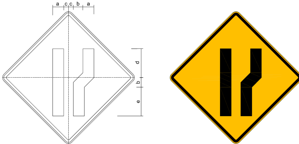
Figura A.89 – Placa A-21e – Alargamento de pista à direita
