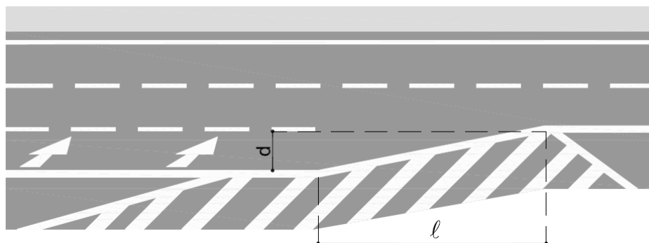
Figura 245 – Marca de transição de largura de pista (MTL)
