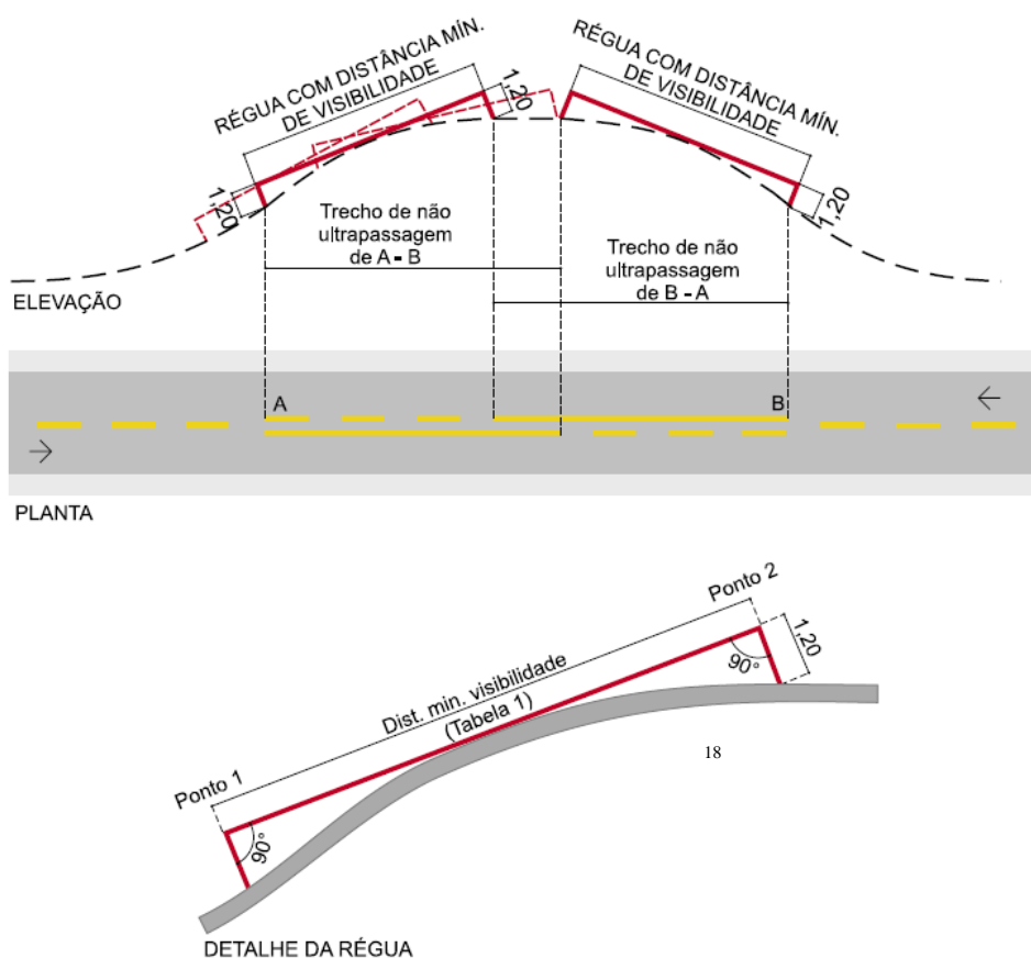
Figura 222 – Distância de visibilidade de ultrapassagem – Vertical
