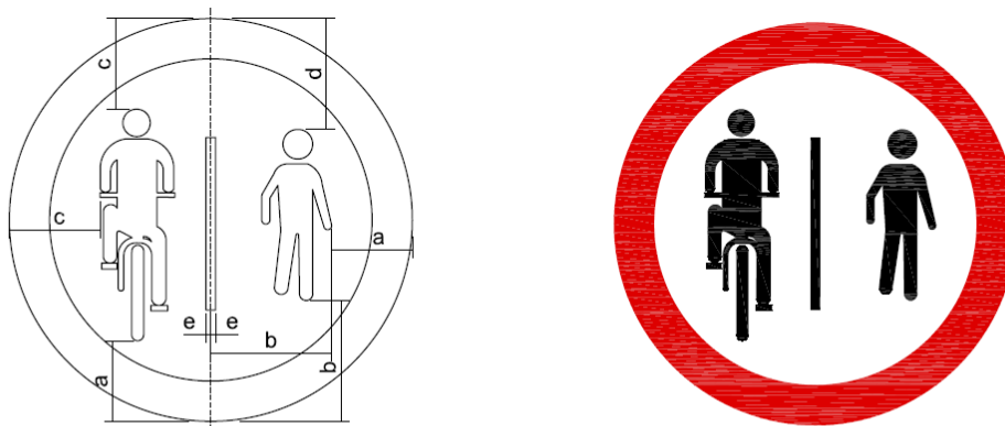
Figura A.48 – Placa R-36a – Ciclistas à esquerda, pedestres à direita
