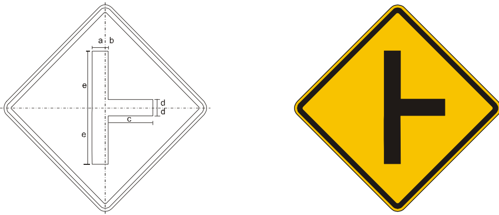
Figura A.67 – Placa A-7b – Via lateral à direita
