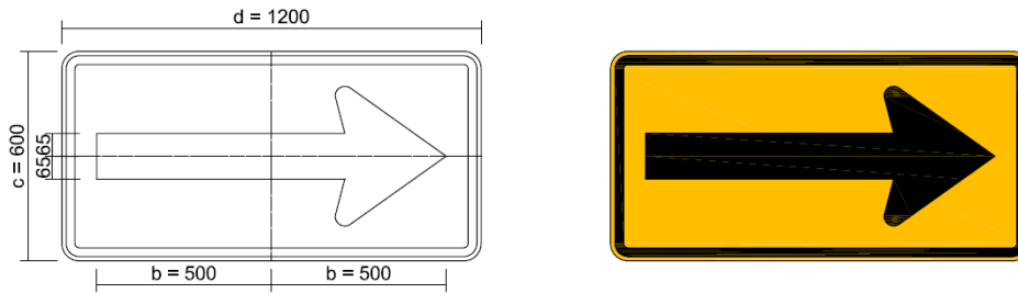
Figura A.93 – Placa A-26a – Sentido único
