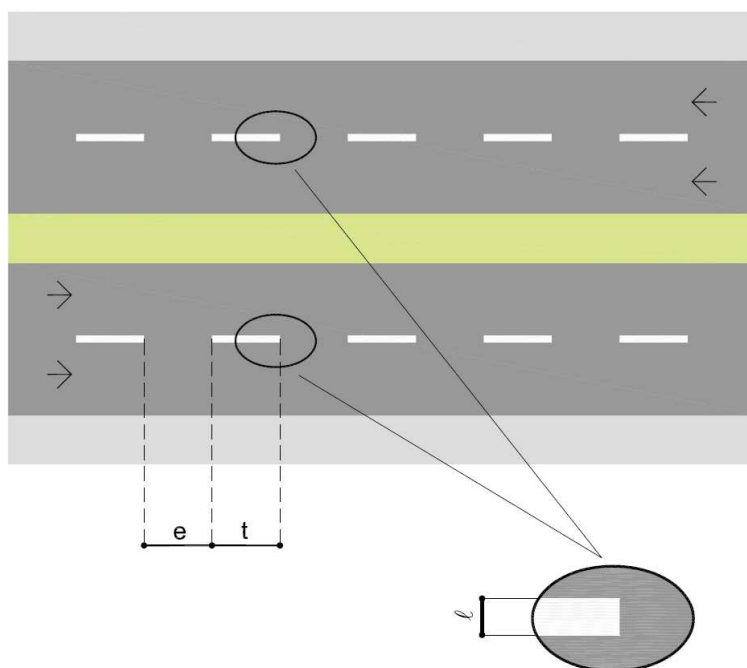
Figura 228 – Linha simples tracejada (LMS-2)
