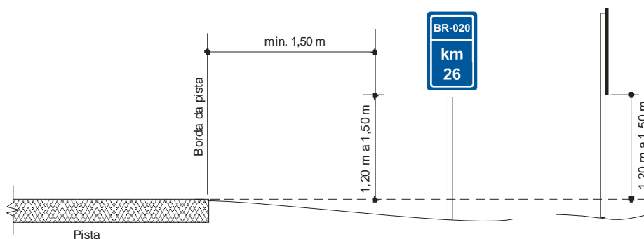
Figura 214 – Posicionamento transversal do sinal de identificação quilométrica
