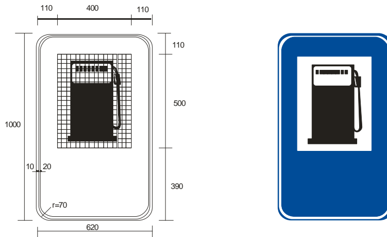
Figura A.122 – Placa I-1 – Abastecimento
