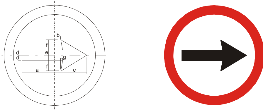
Figura A.31 – Placa R-24a – Sentido de circulação da via/pista
