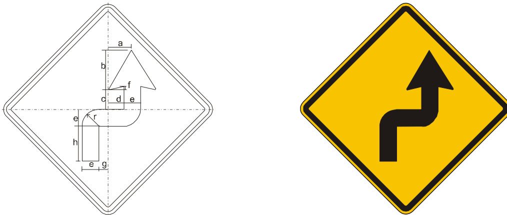
Figura A.62 – Placa A-4b – Curva acentuada em “S” à direita
