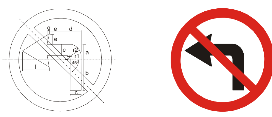
Figura A.6 – Placa R-4a – Proibido virar à esquerda
