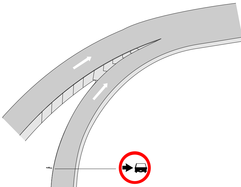
Figura 34 – Entrada de ramo
