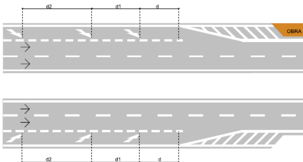
Figura 253 – Exemplo de uso de seta MOF
