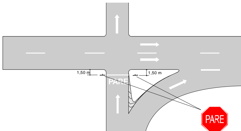
Figura 11 – Aproximação com ilha triangular
