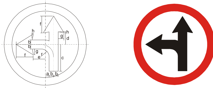
Figura A.35 – Placa R-25c – Siga em frente ou à esquerda
