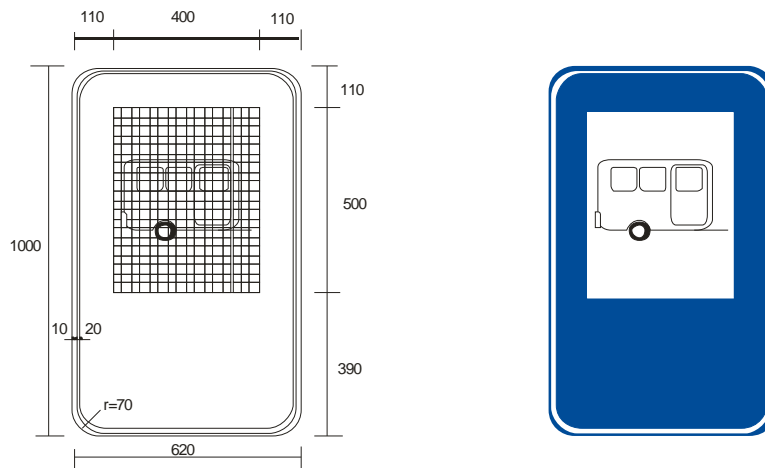
Figura A.133 – Placa I-12 – Ônibus
