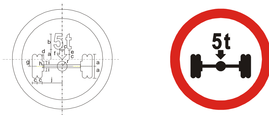
Figura A.24 – Placa R-17 – Peso máximo permitido por eixo
