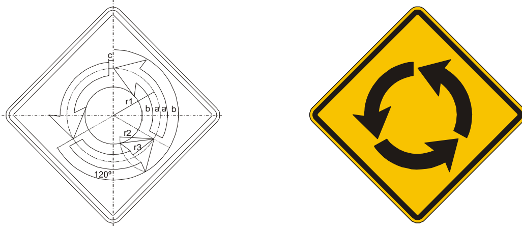
Figura A.74 – Placa A-12 – Interseção em círculo
