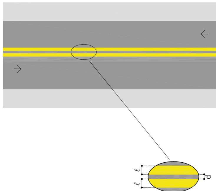
Figura 226 – Linha dupla contínua (LFO-3)
