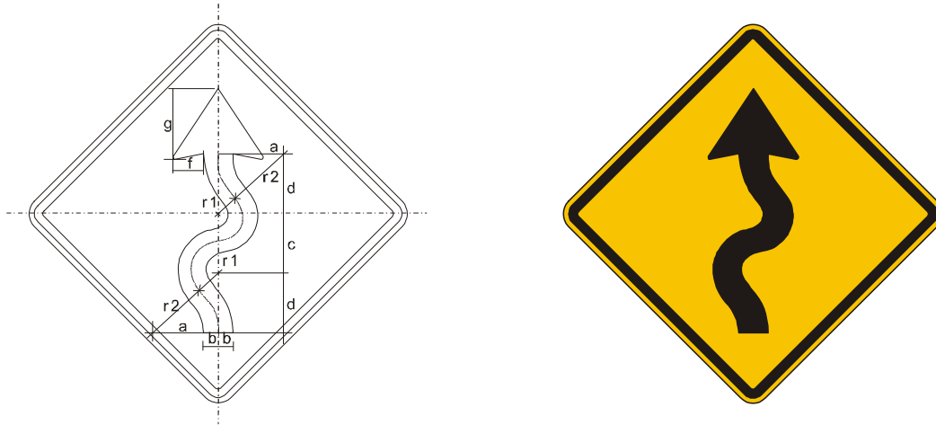
Figura A.59 – Placa A-3a – Pista sinuosa à esquerda
