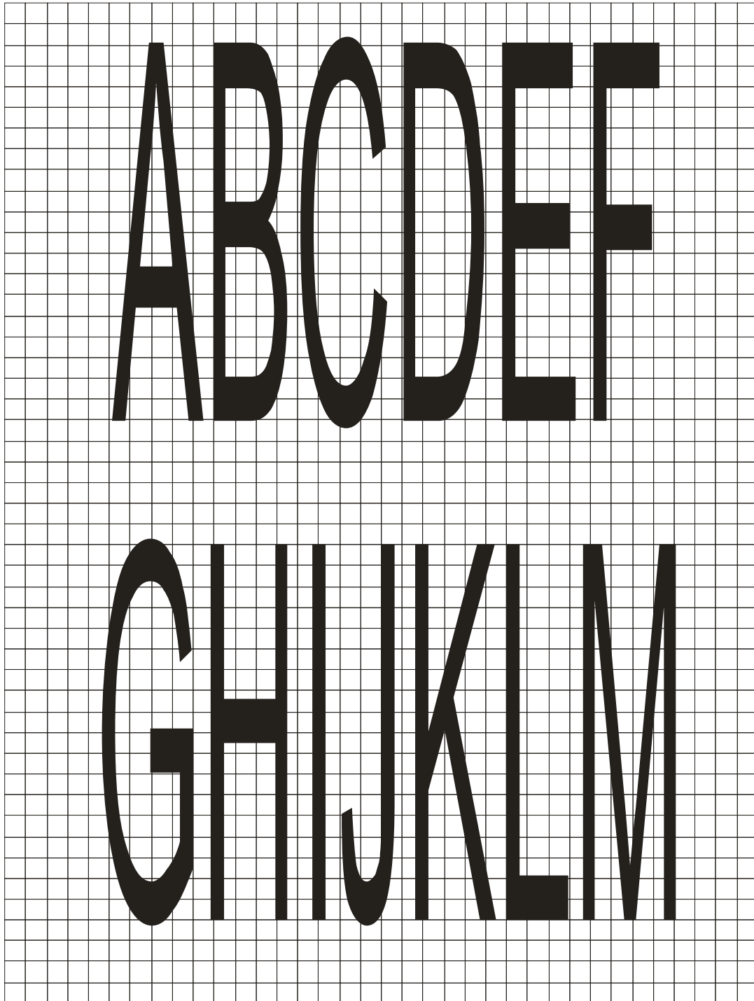
Figura A.146 – Letras A a M – Para V \leq 60 km/h em vias urbanas
