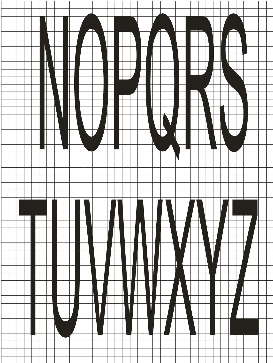
Figura A.147 – Letras N a Z – Para V \leq 60 km/h em vias urbanas
