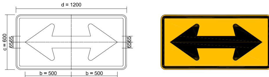
Figura A.94 – Placa A-26b – Sentido duplo
