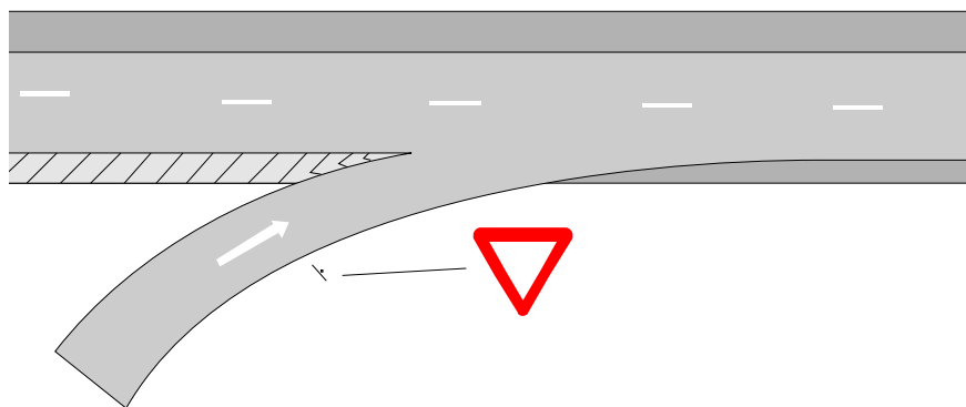
Figura 15 – Ramo de conversão à direita e sem faixa de aceleração
