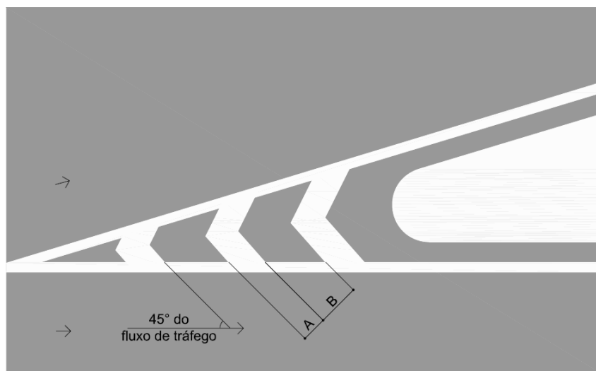
Figura 243 – Marcas de áreas de pavimento não utilizável (MAN)
