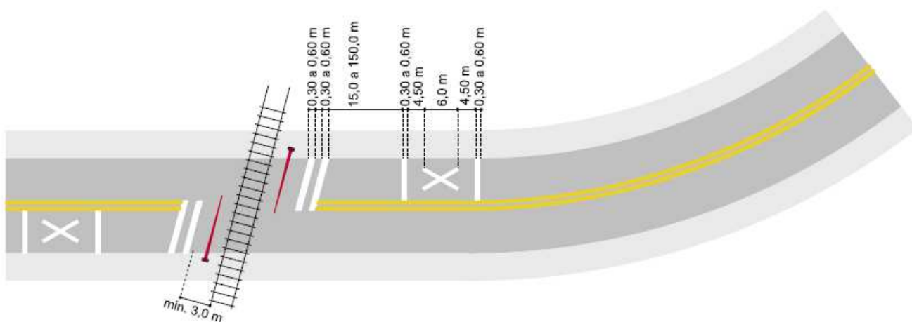
Figura 257 – Exemplo de uso da marca “Cruz de Santo André” em cruzamento rodoferroviário
