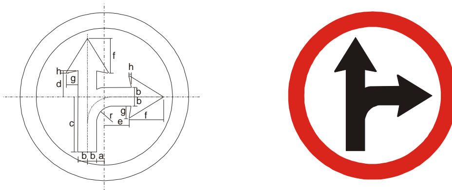
Figura A.36 – Placa R-25d – Siga em frente ou à direita
