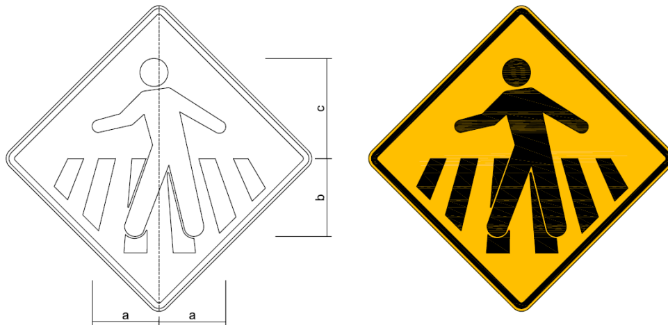
Figura A.103 – Placa A-32b – Passagem sinalizada de pedestres
