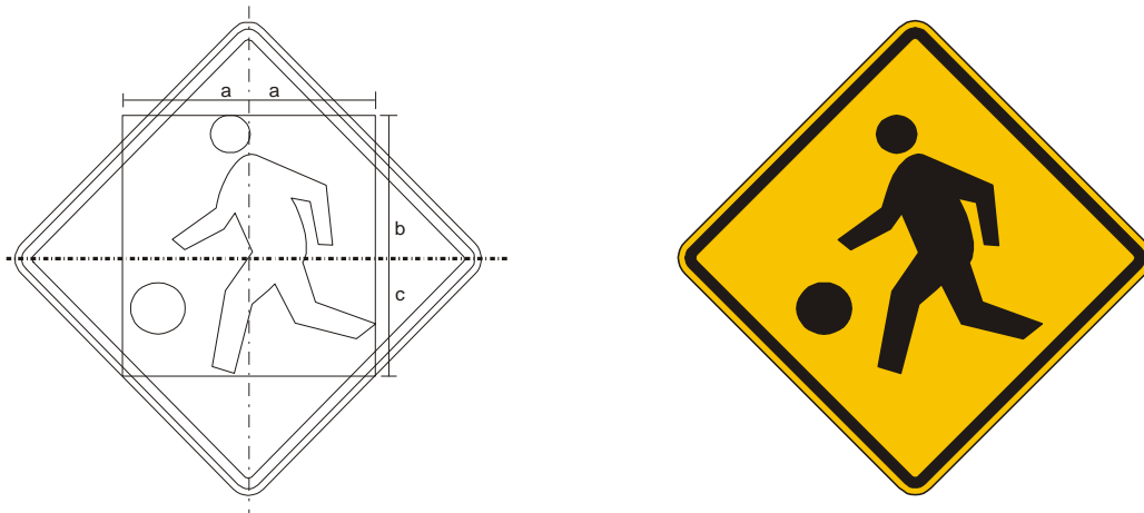
Figura A.106 – Placa A-34 – Crianças
