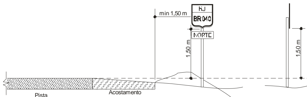
Figura 212 – Seção transversal com o sinal de identificação
