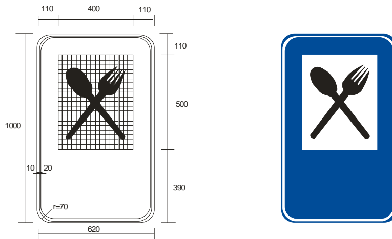
Figura A.123 – Placa I-2 – Restaurante
