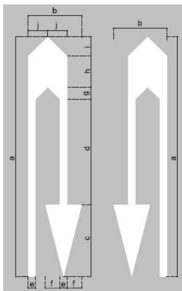
Figura 250 – Setas “retorno à direita” e “retorno à esquerda”
