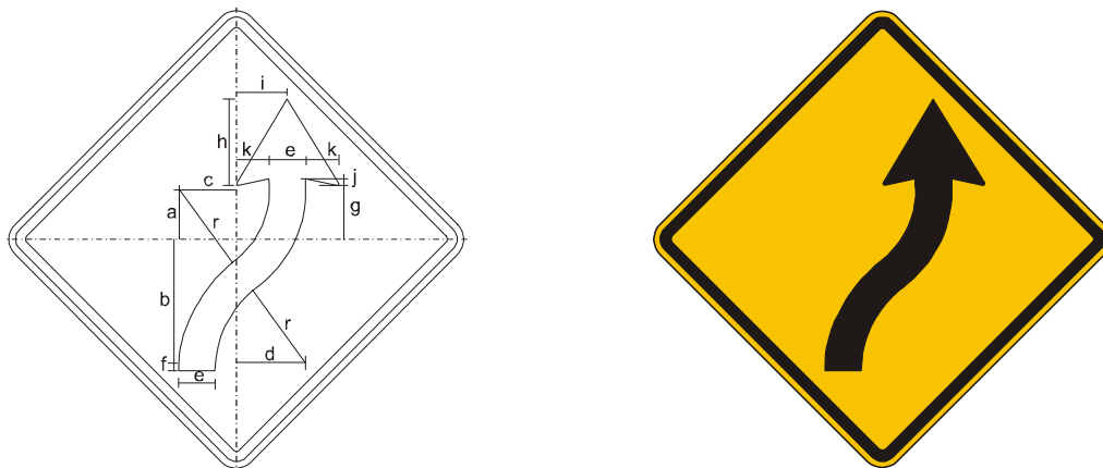
Figura A.64 – Placa A-5b – Curva em “S” à direita
