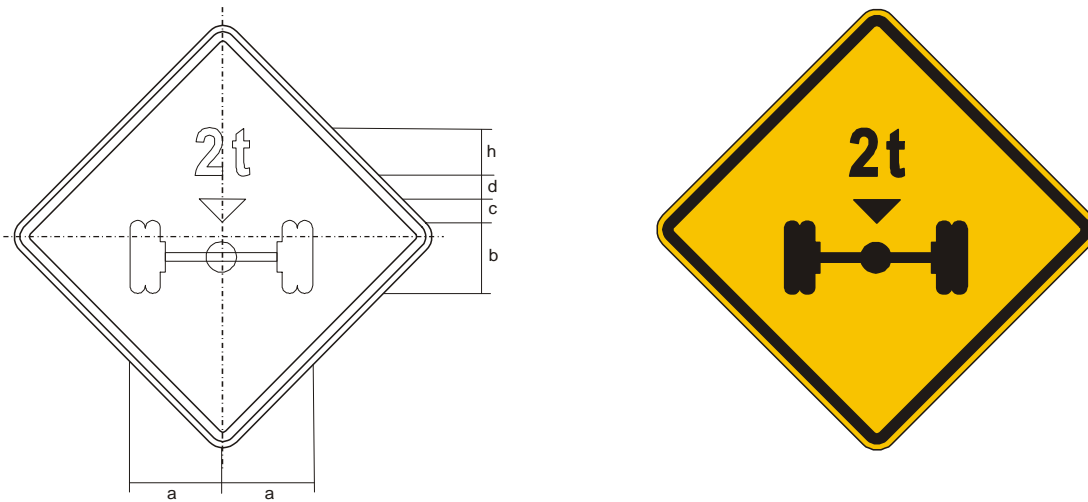
Figura A.120 – Placa A-47 – Peso limitado por eixo
