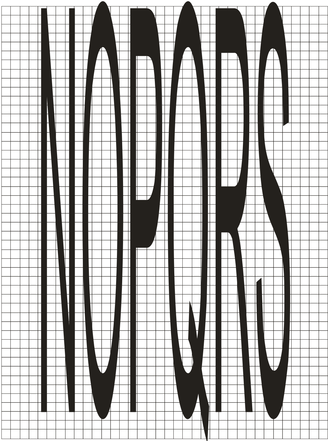
Figura A.157 – Letras N a S – Para V \geq 60 km/h – Vias rurais
